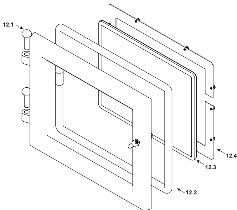
#12 Door Assembly
