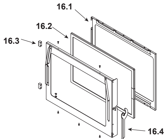
#16 Door Assembly
