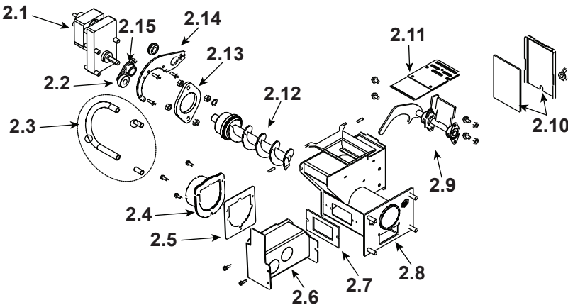
Ensemble du dispositif d'alimentation n° 2
