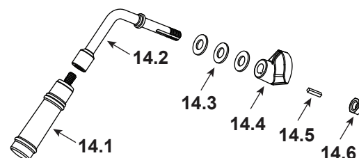
Assemblage pour poignée de porte n° 14
