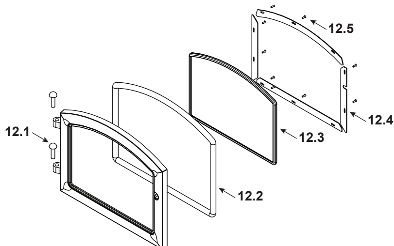
Assemblage de porte n° 12
