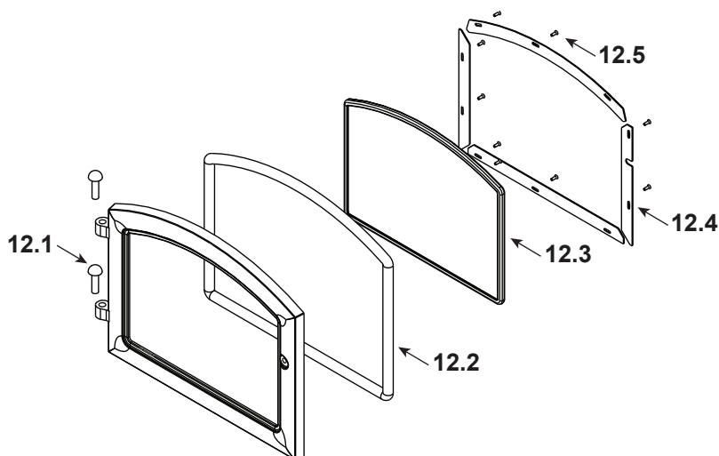
Assemblage pour porte n° 12
