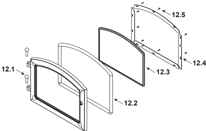
#12 Door Assembly
