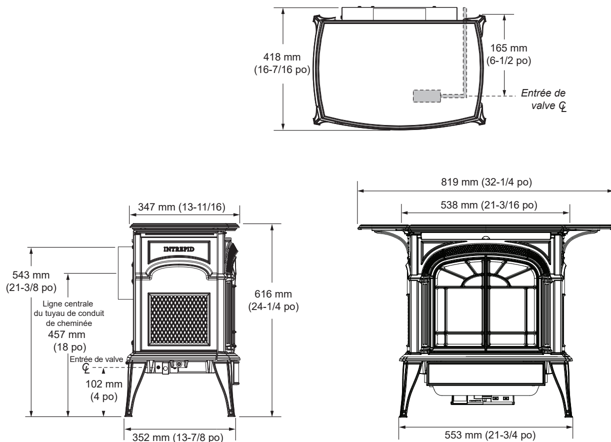
Figure 2.1 – Dimensions de l'Intrepid DV.
