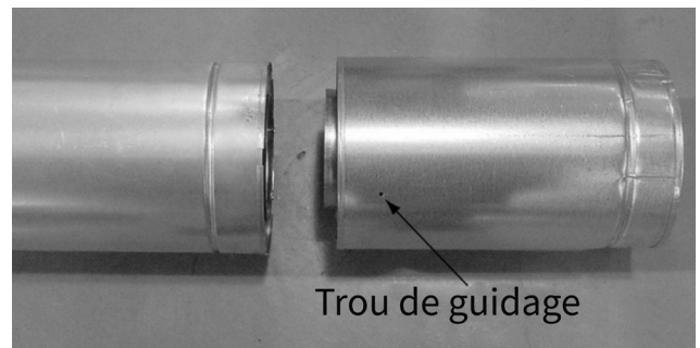
Figure 3.3 – Trous de guidage de la section coulissante
