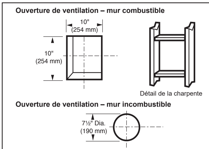
Figure 3.10 – Localiser l'ouverture de la ventilation sur le mur
