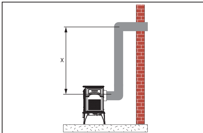
Figure 3.11 – Exigences quant à la hauteur verticale
