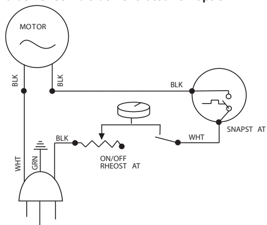
Figure 6.2 – Circuit du ventilateur
