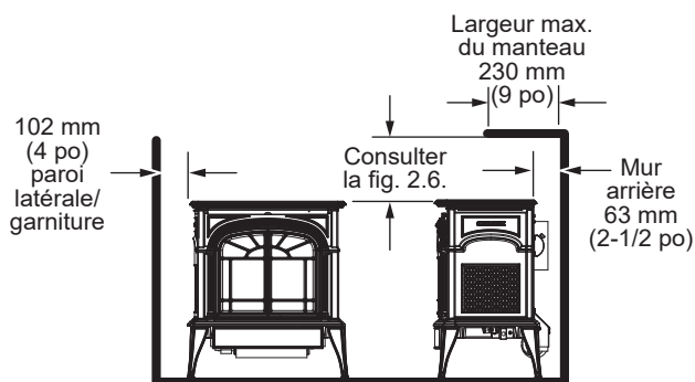
Figure 2.5 – Dégagements avec le mur et le plafond.
