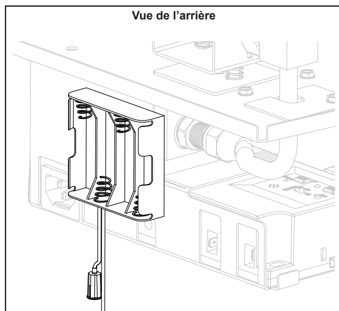
Figure 4.5 – Boîtier de piles
