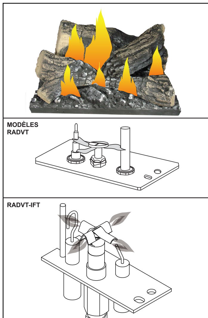
Figure 4.6 – Apparence correcte des flammes de la veilleuse et du brûleur.
