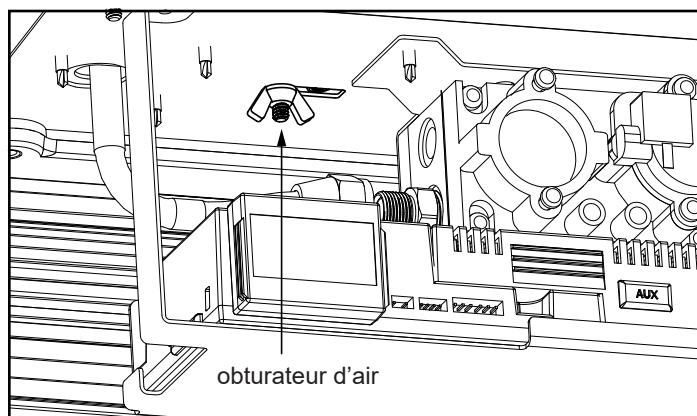
Figure 4.7 - obturateur d'air
