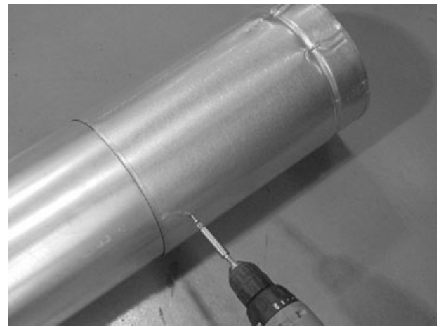
Figure 3.5 – Vis dans la section coulissante
