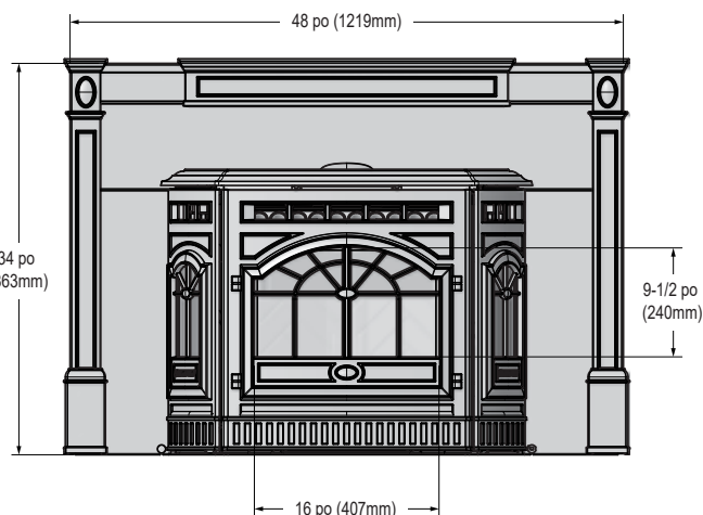
Figure 8.6 - Vue de face avec grand ensemble Surround et Cast Panel
