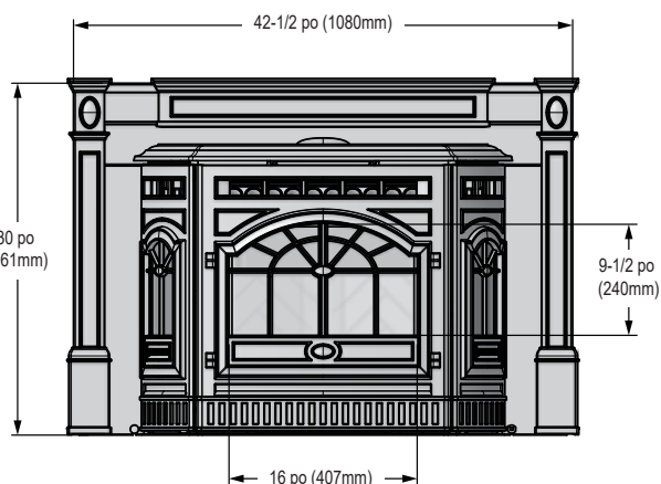
Figure 8.5 - Vue avant avec petit ensemble Surround et Cast Panel
