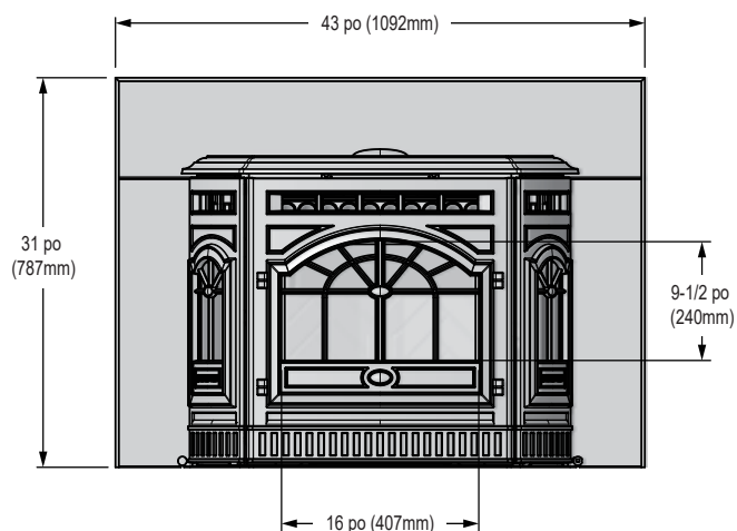
Figure 8.2 - Vue avant avec petit ensemble de panneaux surround
