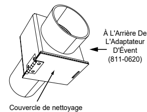
Figure 21.3 – Adaptateur de ventilation arrière
