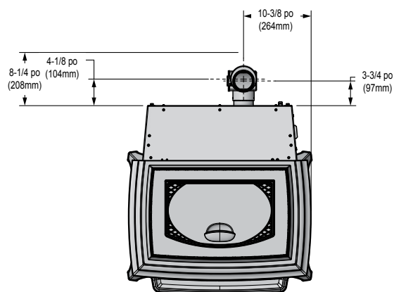
Figure 8.5 - Vue de dessus avec adaptateur de ventilation supérieure (TPVNT-6) et adaptateur de décalage (811-0720).
