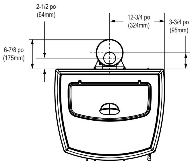
Figure 8.3 - Vue de dessus avec adaptateur supérieur de ventilation (TPVNT-2) et adaptateur de dévoiement (812-3570).
