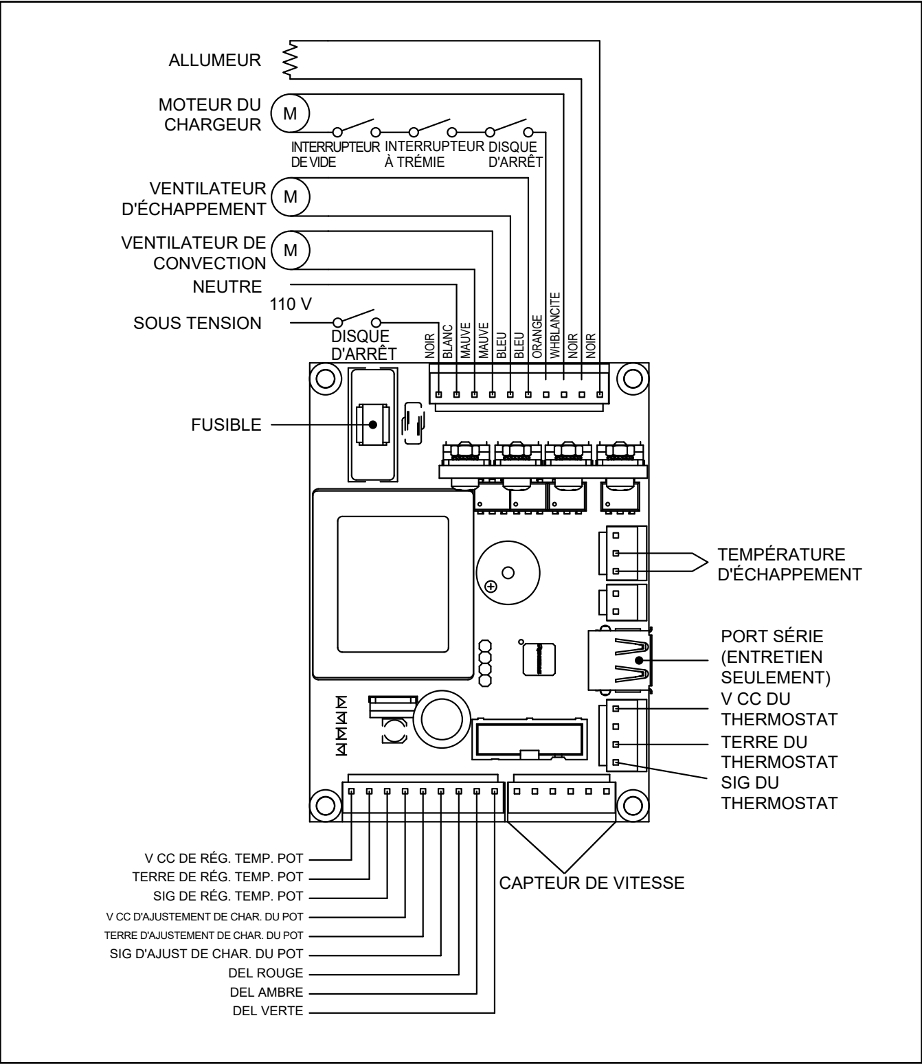
Schéma de câblage du panneau de commande
