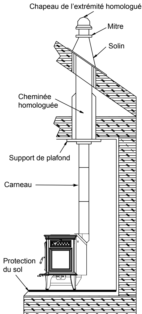
Figure 14.1 - Cheminée préfabriquée pour l'intérieur
