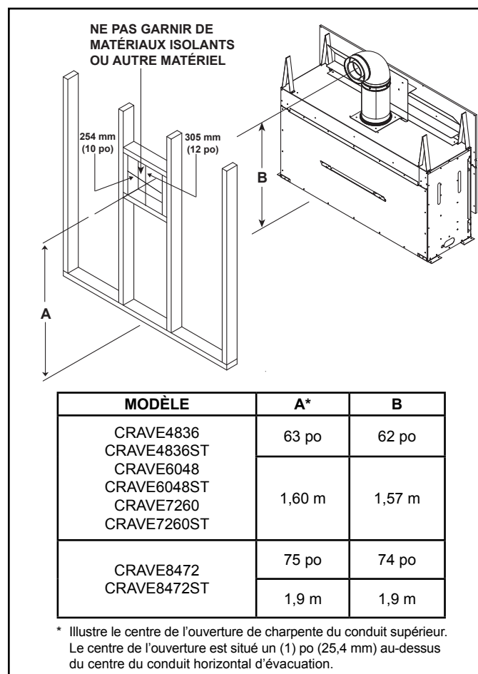
Figure 5.2 Pénétration du mur
