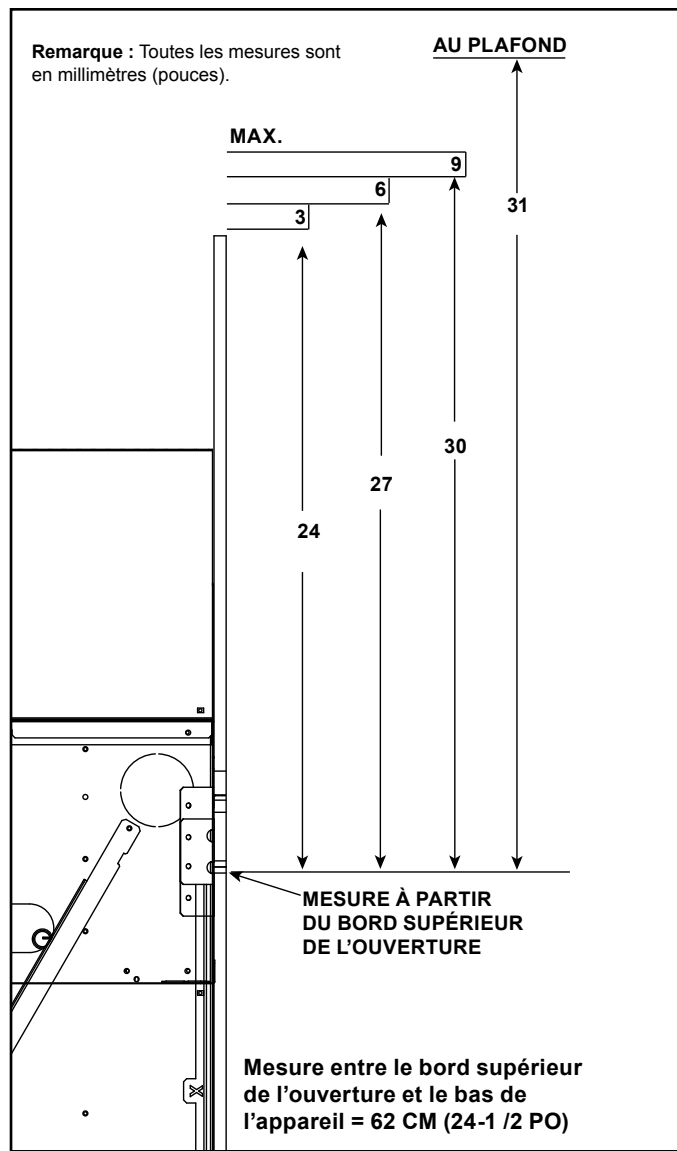
Figure 10.11 Minimum vertical et maximum horizontal Dimensions des matériaux inflammables - CRAVE7260 et CRAVE8472
