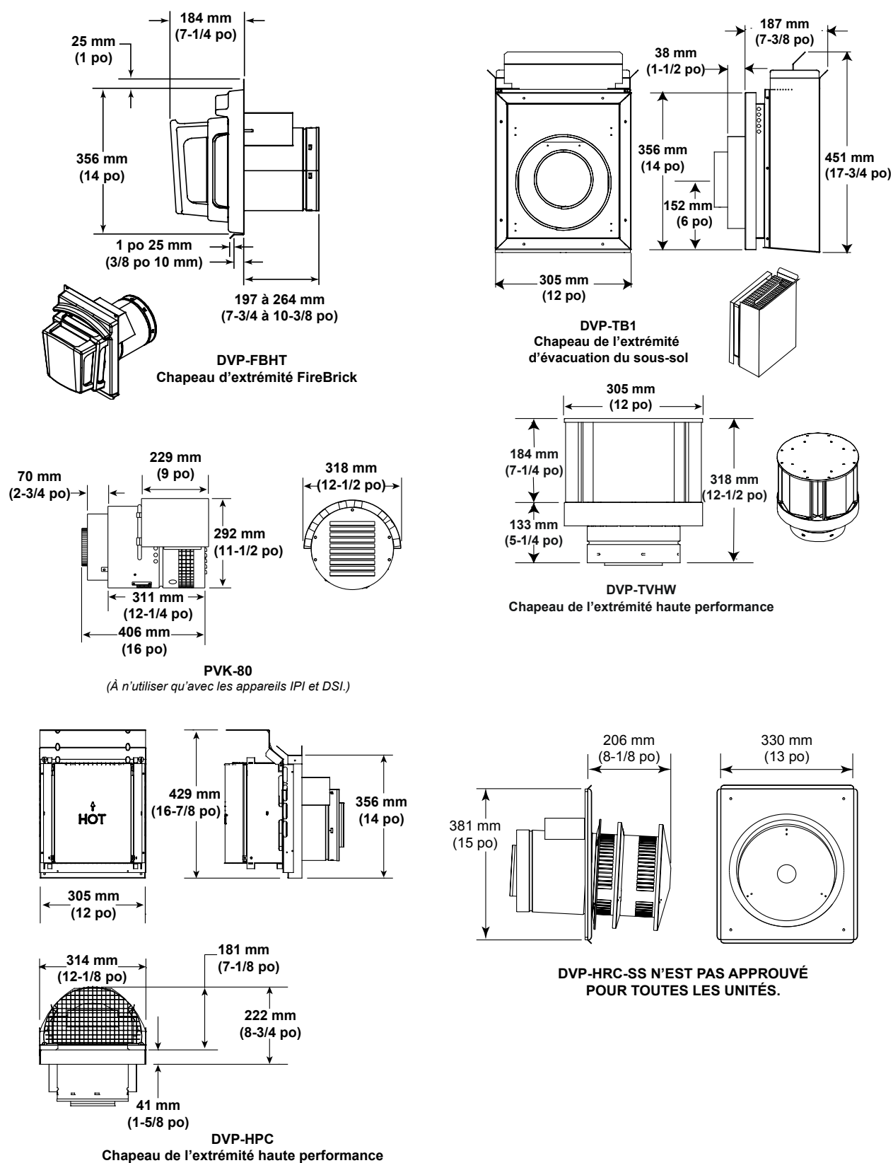
Figure 12.4 Composants du conduit DVP
