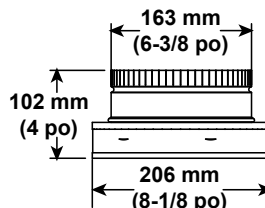
SLP-LPC Chapeau SLP à profil bas
