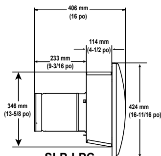
SLP-LPC Chapeau SLP à profil bas
