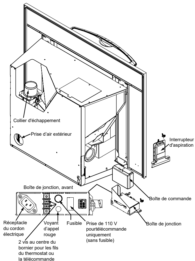
Figure 30.4 – Emplacements des composants - Côté gauche
