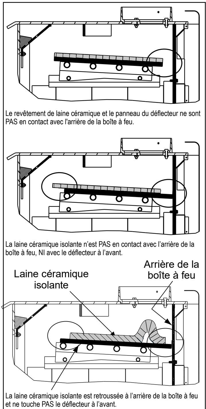
Figure 19.2 - Mauvais positionnement du déflecteur et de la laine céramique
