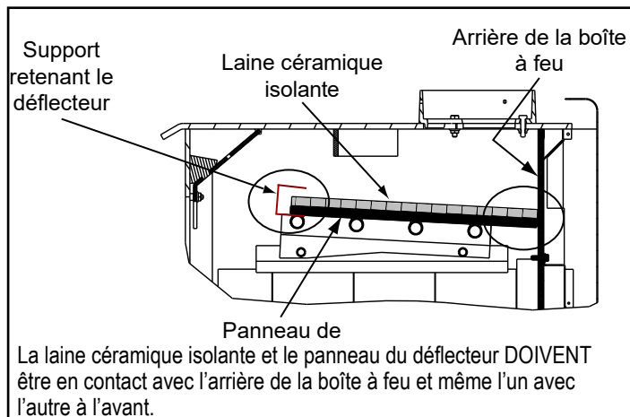
Figure 19.1 - Bon positionnement du déflecteur et de la laine céramique
