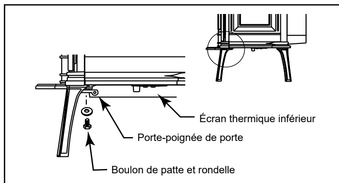
Figure 5.4 - Positions du porte-poignée et de l'écran thermique.
