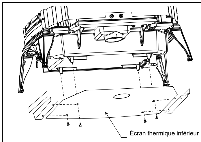
Figure 5.5 - Fixation de l'écran thermique inférieur.
