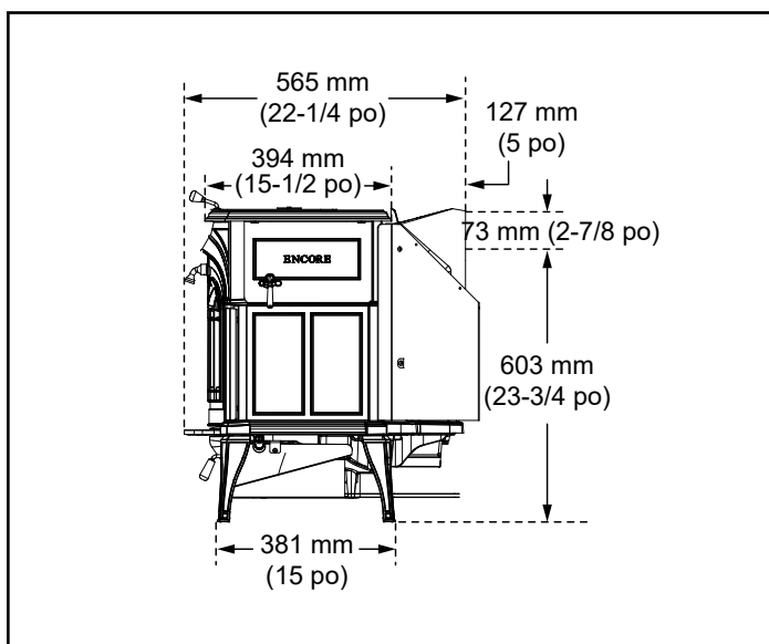
Figure 3.2 – Vue latérale
