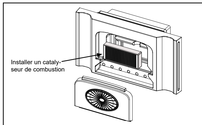
Figure 5.10 - Installer un catalyseur de combustion.
