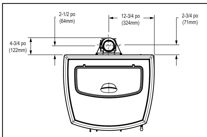
Figure 8.2 - Vue de dessus avec adaptateur supérieur de ventilation (TPVNT-2) et adaptateur de dévoiement (811-0720).
