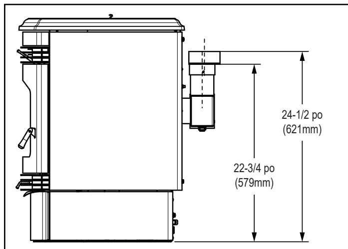
Figure 9.4 - Vue latérale avec adaptateur supérieur de ventilation (TPVNT-6) et adaptateur de dévoiement (811-0720).
