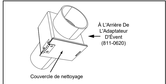
Figure 21.3 - Arrière Adaptateur de ventilation
