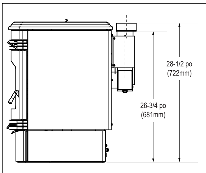
Figure 9.2 - Vue latérale avec adaptateur supérieur de ventilation (TPVNT-2) et adaptateur de dévoiement (811-0720).
