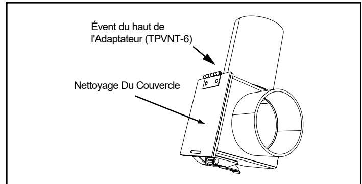
Figure 21.4 – L'arrière à l'adaptateur supérieur de ventilation – 90°
