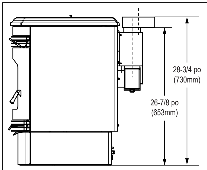
Figure 9.3 - Vue latérale avec adaptateur supérieur de ventilation (TPVNT-2) et adaptateur de dévoiement (812-3570).
