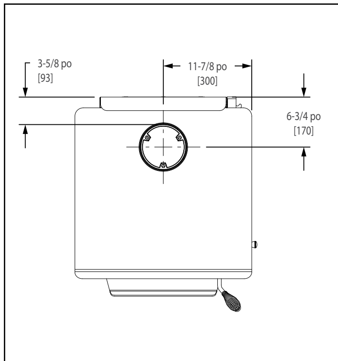
Figure 8.2 - Vue de dessus
