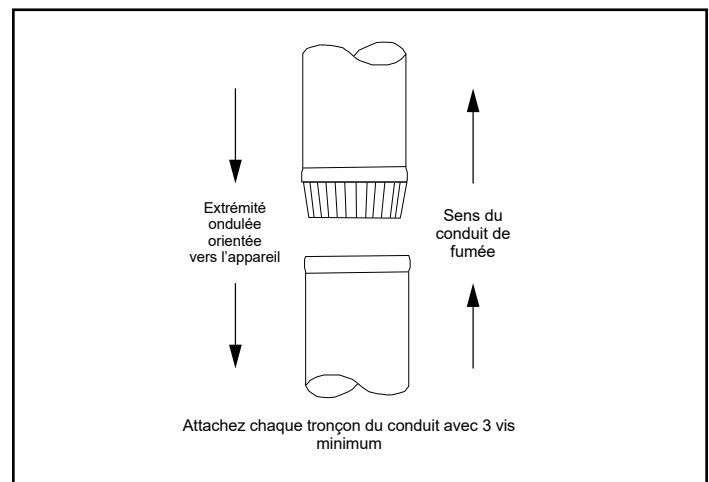
Figure 15.3 - Carneau (tuyau d'appareil)
