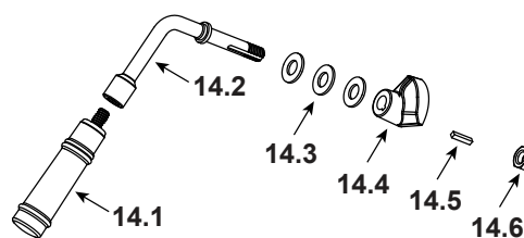
Assemblage pour poignée de porte n° 14
