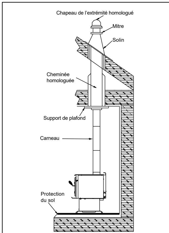
Figure 16.1 - Cheminée préfabriquée pour l'intérieur
