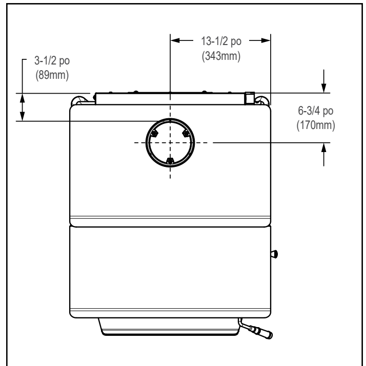
Figure 9.2 - Vue de dessus
