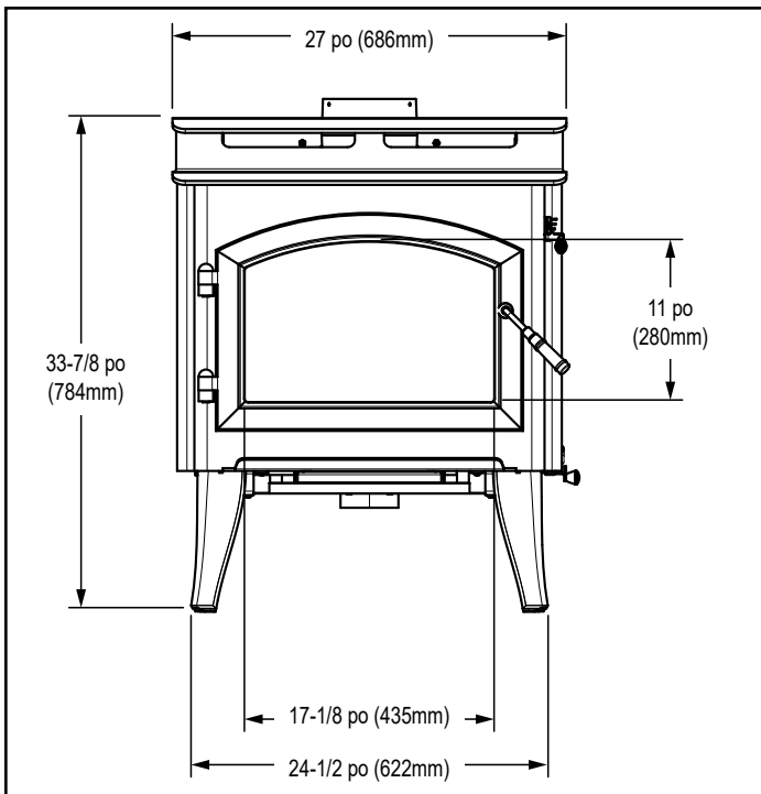
Figure 10.1 – Vue avant
