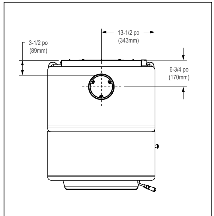
Figure 10.3 - Vue de dessus
