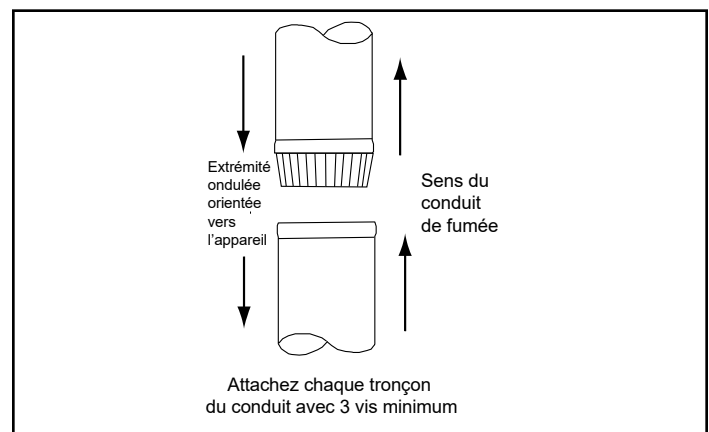
Figure 17.3 - Carneau (tuyau d'appareil)
