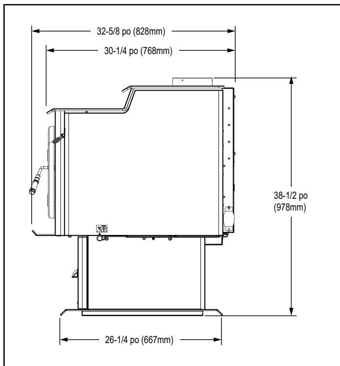
Figure 8.3 - Vue latérale
