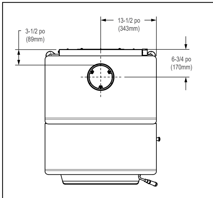
Figure 8.2 - Vue de dessus
