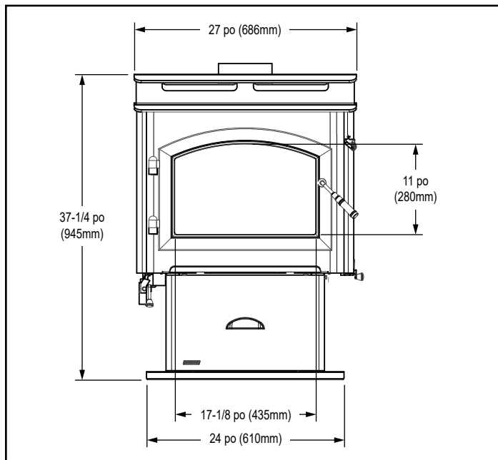
Figure 8.1 - Vue avant
