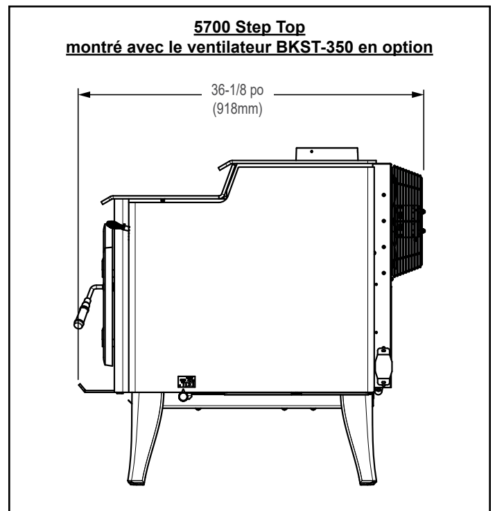
Figure 10.4 – Vue latérale avec option de soufflante TRAD-LEG et BKST-350.
