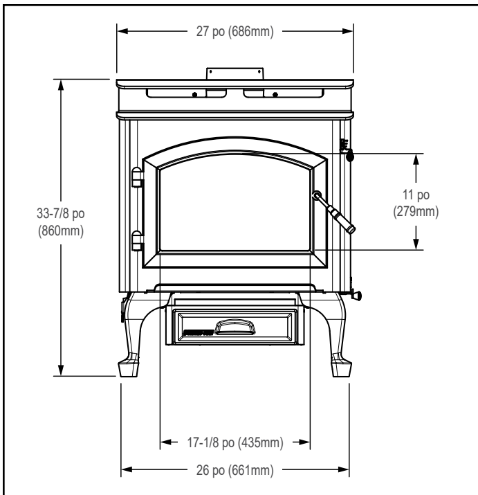
Figure 9.1 – Vue avant
