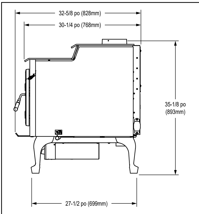
Figure 9.3 – Vue latérale
