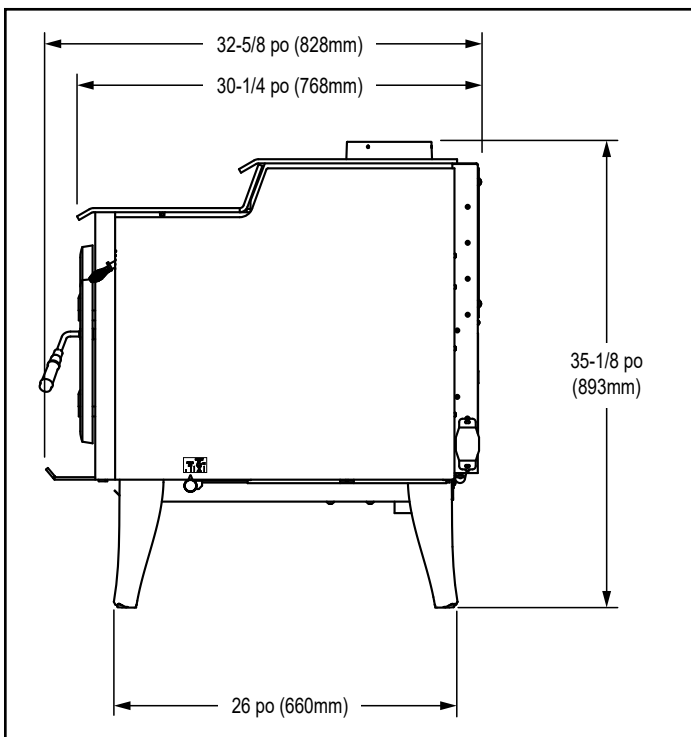
Figure 10.2 – Vue latérale
