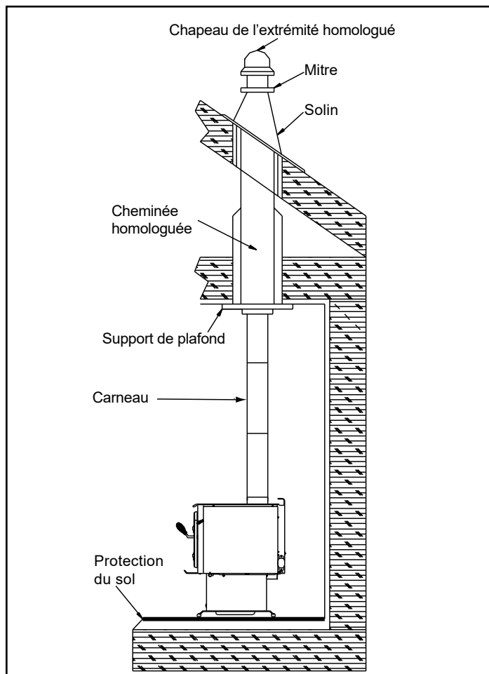
Figure 14.1 - Cheminée préfabriquée pour l'intérieur
