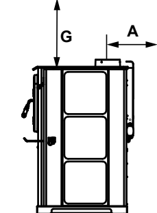
VUE LATÉRALE DE L'ALCÔVE
