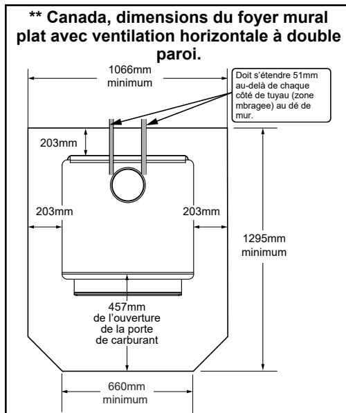
Figure 9.2 - ** Cette dimension varie en fonction de l'installation.
