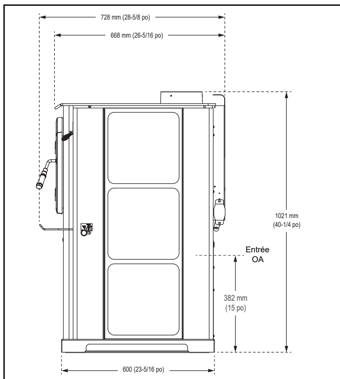
Figure 8.3 - Vue latérale
