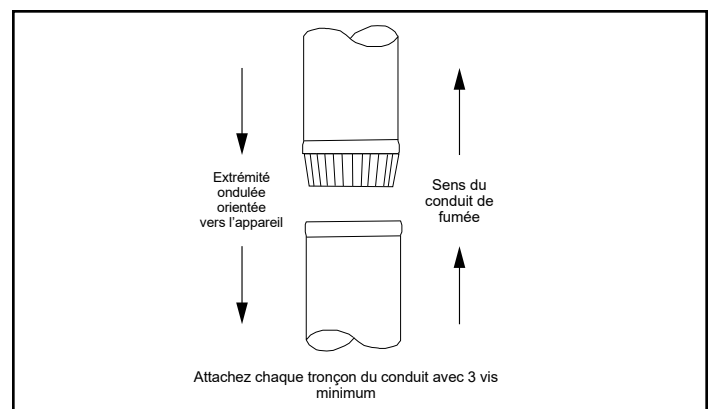
Figure 15.3 - Carneau (tuyau d'appareil)
