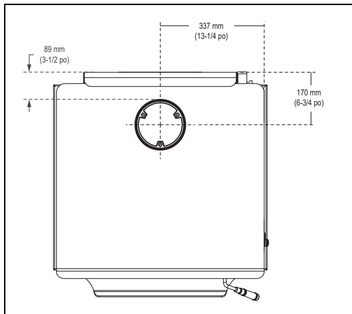
Figure 8.2 - Vue de dessus
