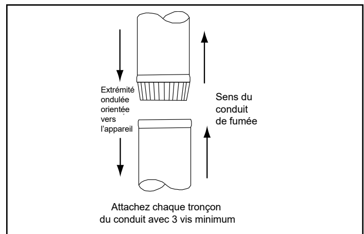
Figure 15.3 - Carneau (tuyau d'appareil)
