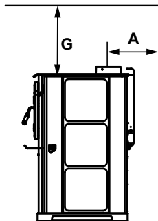
VUE LATÉRALE DE L'ALCÔVE
