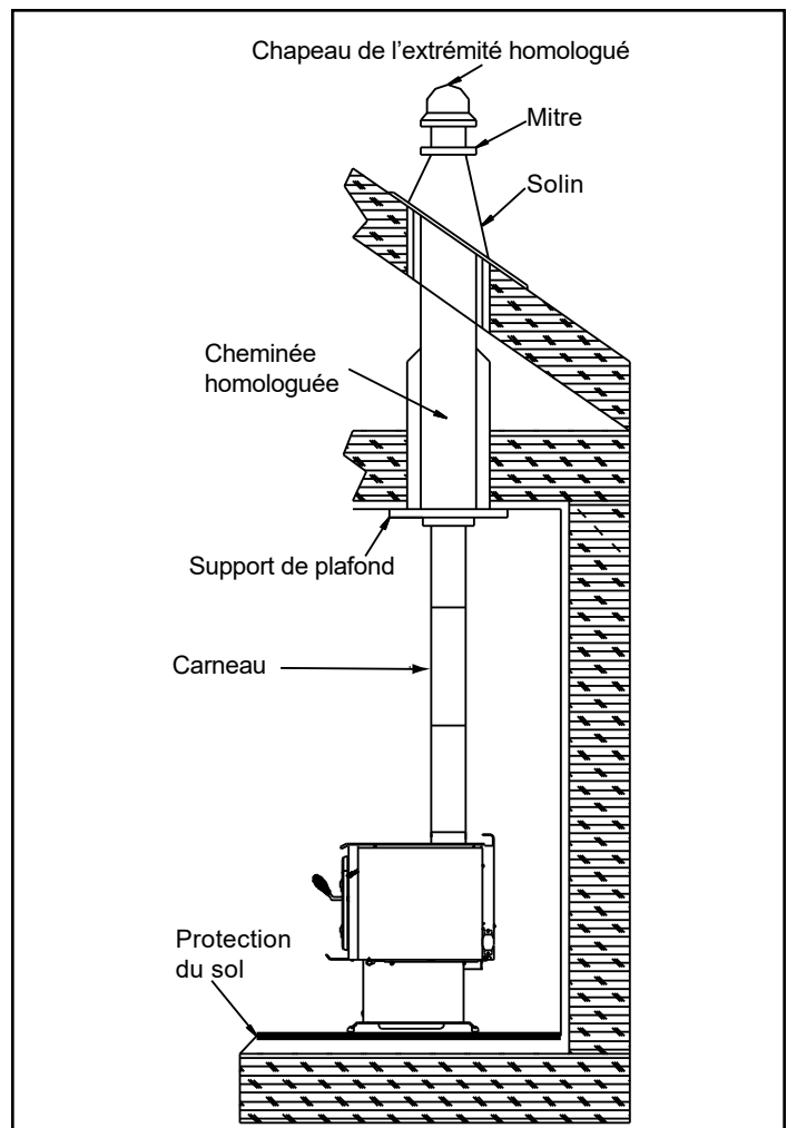
Figure 14.1 - Cheminée préfabriquée pour l'intérieur
