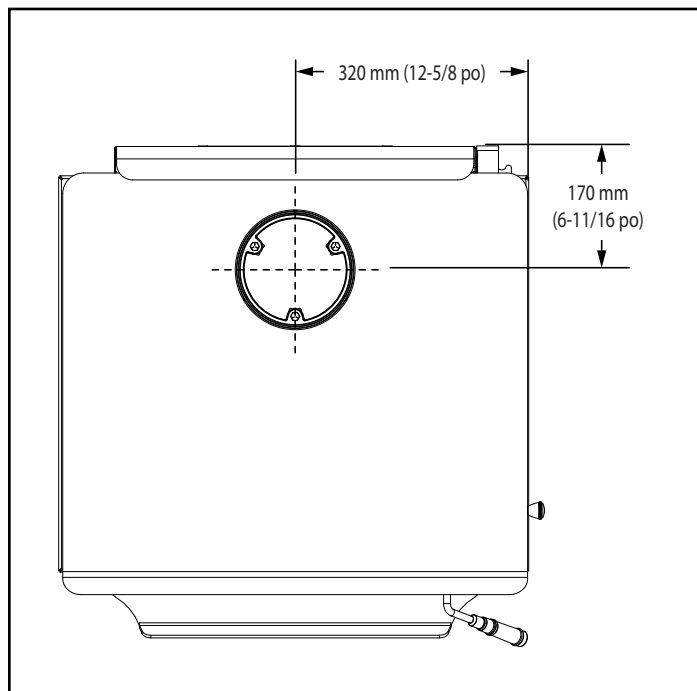
Figure 8.2 - Vue de dessus
