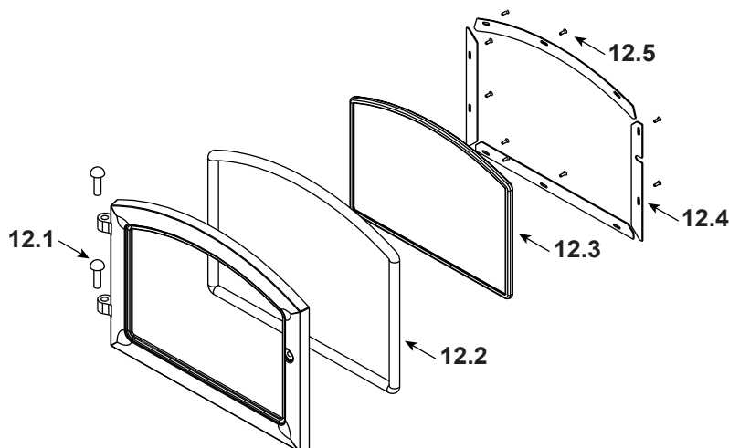
Assemblage pour porte n° 12
