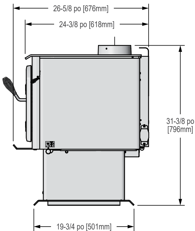
Figure 8.3 - Vue latérale
