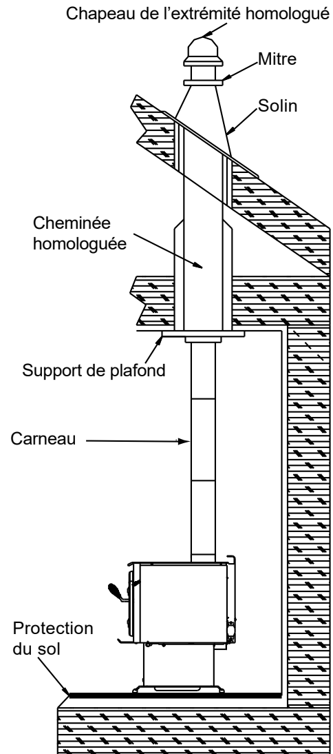
Figure 14.1 - Cheminée préfabriquée pour l'intérieur
