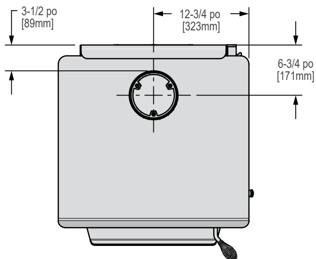
Figure 8.2 - Vue de dessus
