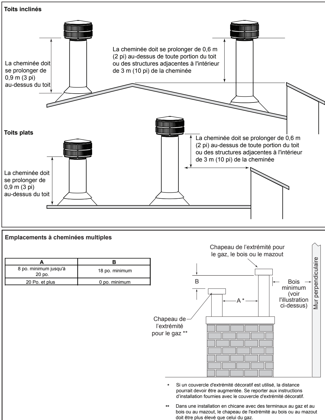
Figure 5.3 Emplacements à cheminées multiples
