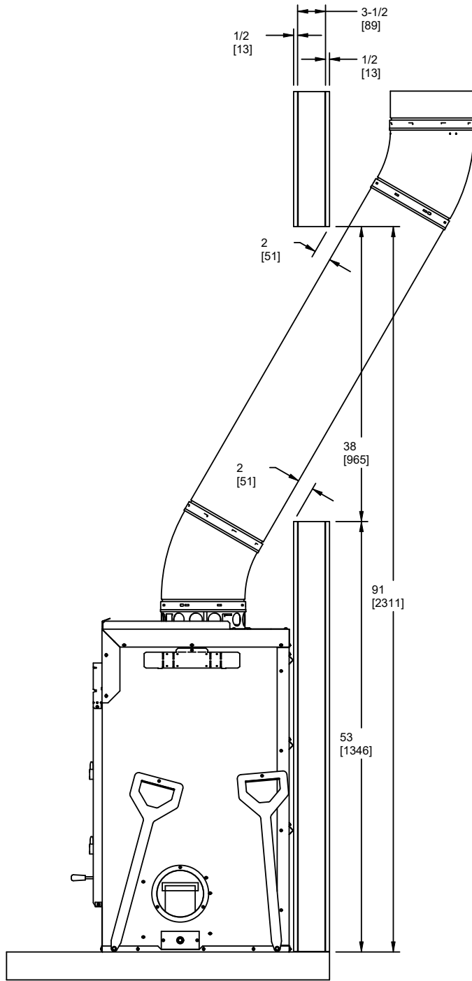
Dévoisement pour une construction murale 2x4
