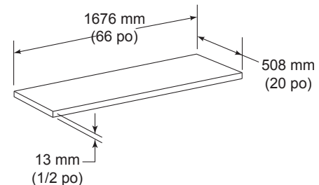
HX4 Prolongement de l'âtre Micore
