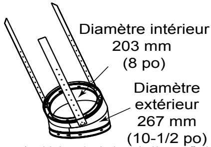
SL315 Dévoisement/conduit de reprise de cheminée- Hauteur effective 380 mm (13-3/8 po) Dévoisement/conduit de reprise de cheminée SL330 - Hauteur effective 394 mm (15-1/2 po)
