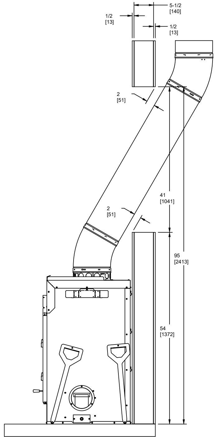
Dévoisement pour une construction murale 2x6
