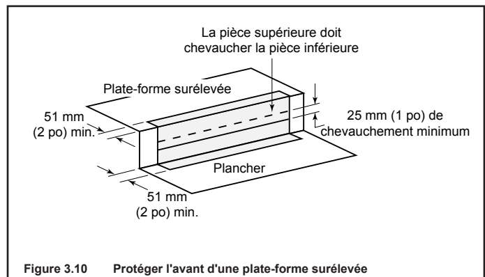
Figure 3.10 Protéger l'avant d'une plate-forme surélevée
