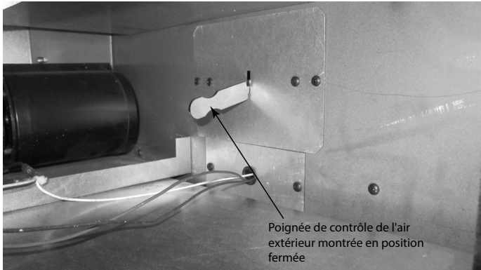
Figure 3.20 Poignée d'air extérieure illustrée sur le côté droit
