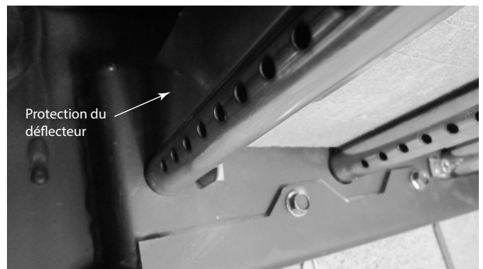
Figure 4.9 Réinstaller le canal de protection du déflecteur
