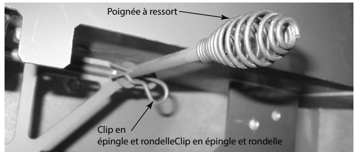
Figure 4.28 Démontage de la poignée à ressort
