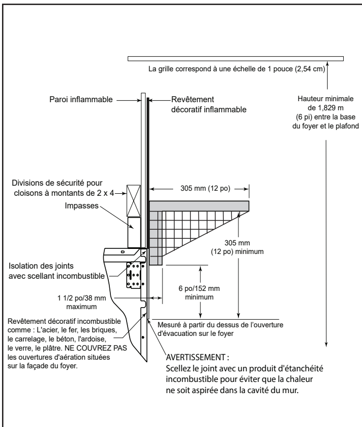
Figure 7.10 Spécifications du manteau de foyer
