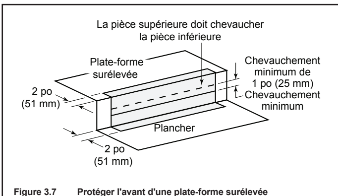
Figure 3.7 Protéger l'avant d'une plate-forme surélevée
