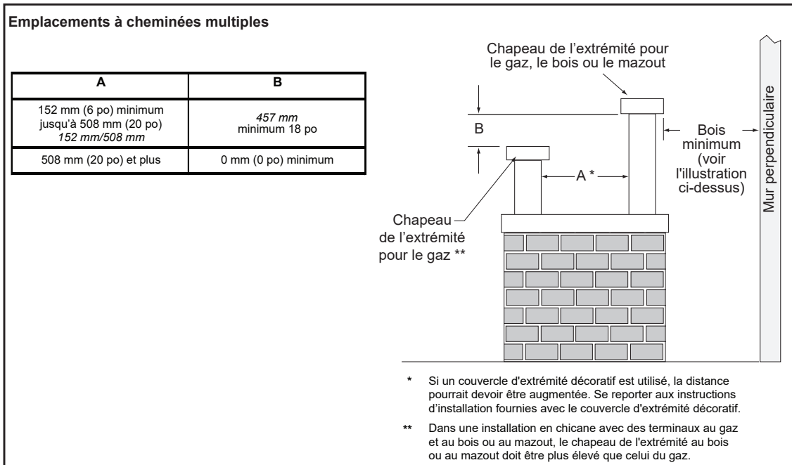
Figure 4.3 Emplacements à cheminées multiples
