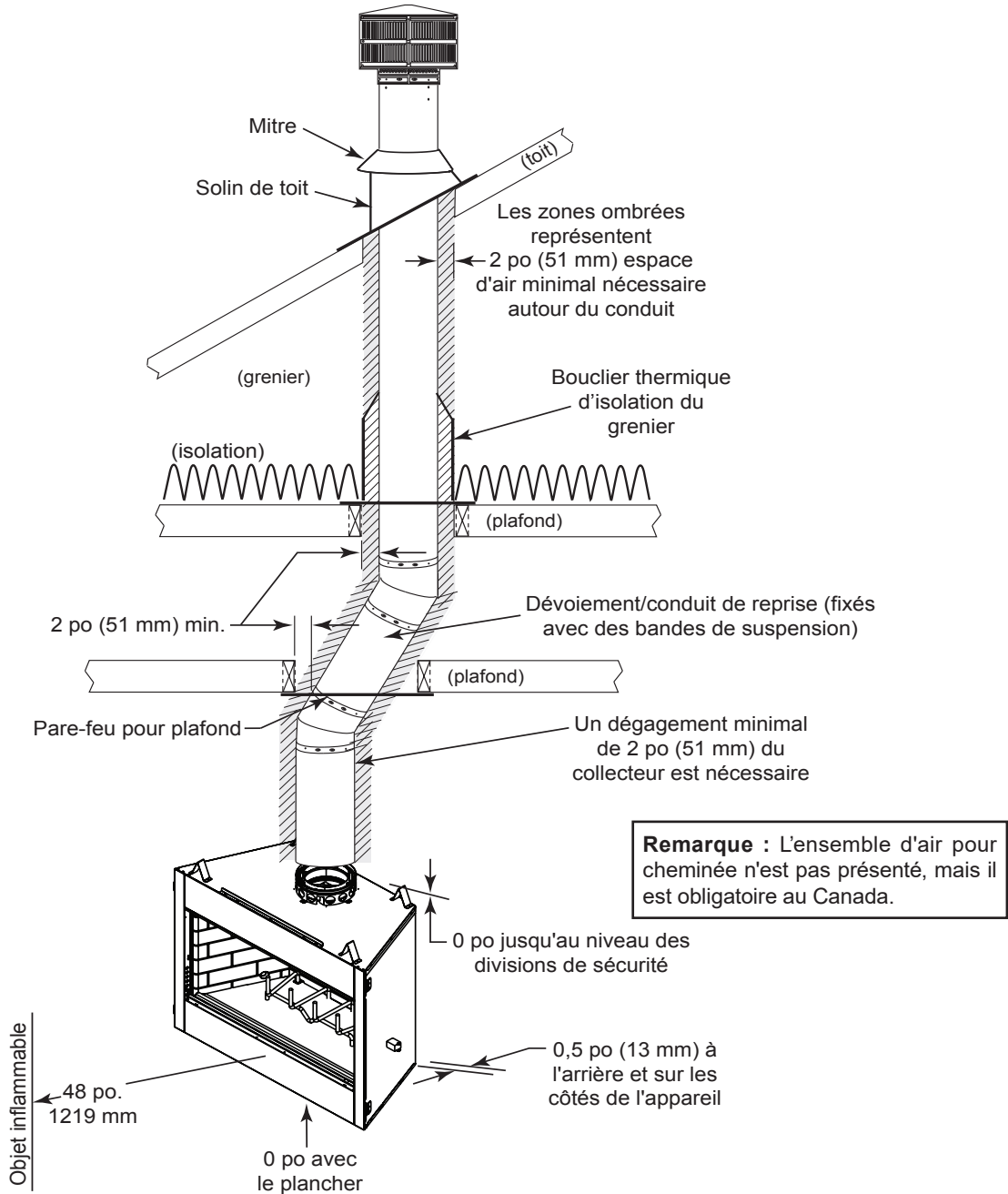
Figure 3.2 Dégagements par rapport aux matériaux inflammables
