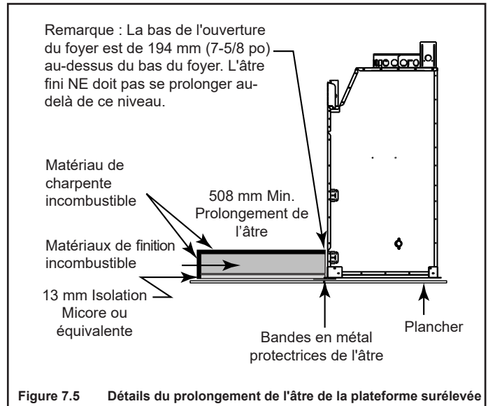
Figure 7.5 Détails du prolongement de l'âtre de la plateforme surélevée
