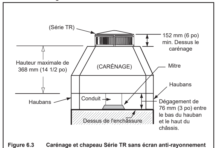
Figure 6.3 Carénage et chapeau Série TR sans écran anti-rayonnement
