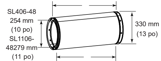
Sections de cheminée
