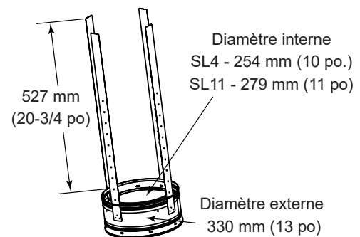
Stabilisateur de cheminée SL11/SL4
