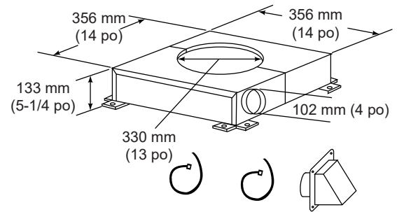
Ensemble de prise d'air extérieur CAK5A
