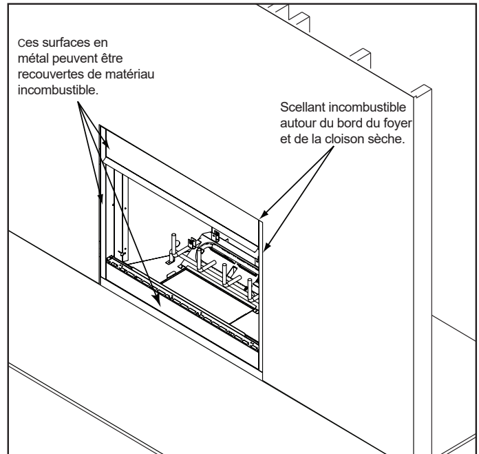
Figure 7.1 Revêtement incombustible
