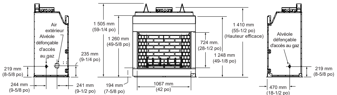
Figure 3.1 Dimensions de l'appareil
