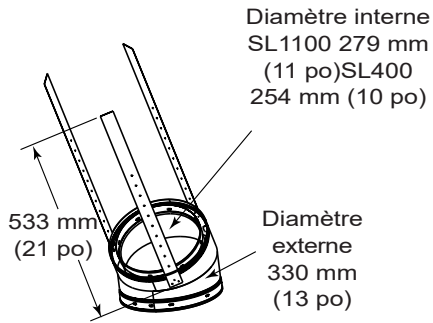
Dévoiemnts/conduits de reprise SL1130/SL430
