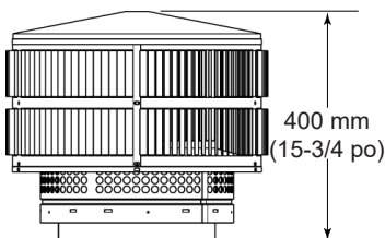
TR11/TR444 - Chapeau de l'extrémité rond
