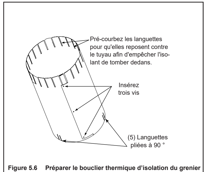
Figure 5.6 Préparer le bouclier thermique d'isolation du grenier
