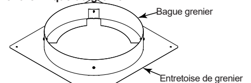
Ensemble du bouclier thermique du grenier
