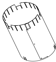
Diamètre une fois assemblé : 432 mm/17 po Hauteur : 610 mm/24 po
