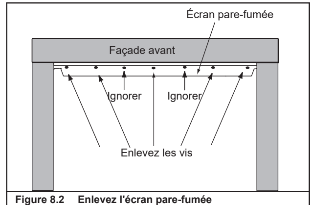
Figure 8.2 Enlevez l'écran pare-fumée
