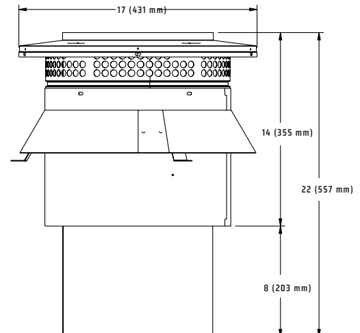
CT11-Adaptateur A
