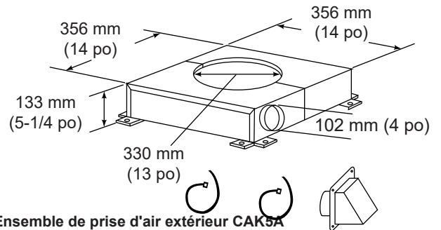
Ensemble de prise d'air extérieur CAK5A
