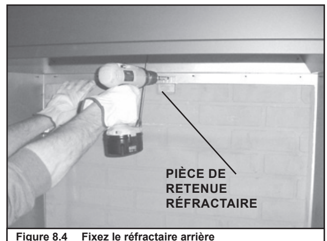
Figure 8.4 Fixez le réfractaire arrière
