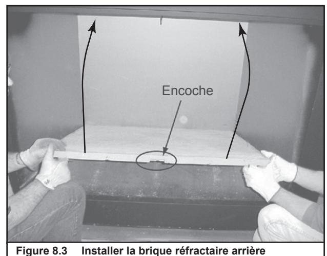
Figure 8.3 Installer la brique réfractaire arrière
