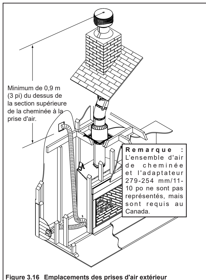
Figure 3.16 Emplacements des prises d'air extérieur
