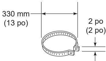
JB577 Bande de jonction de cheminée
