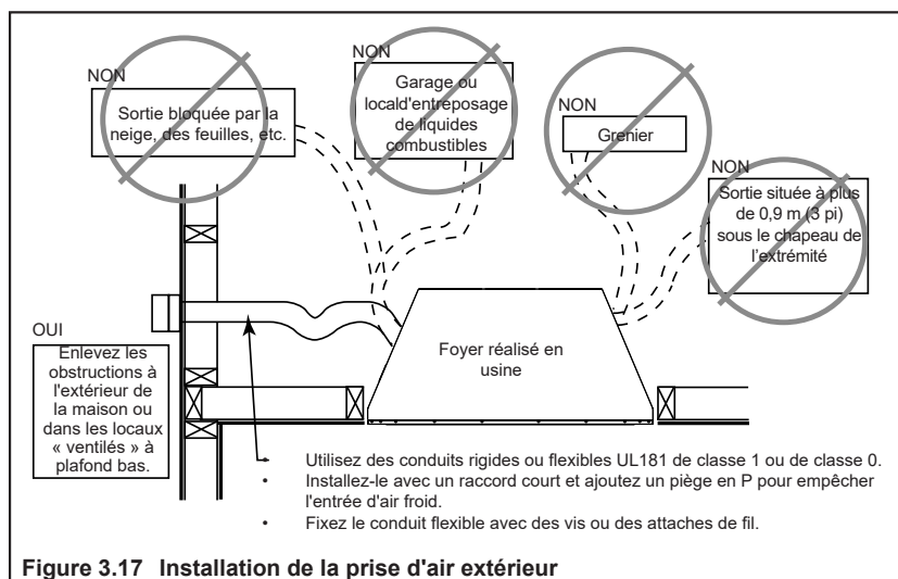
Figure 3.17 Installation de la prise d'air extérieur
