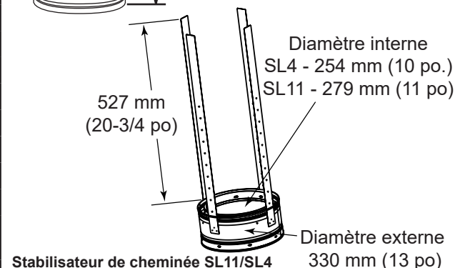
Stabilisateur de cheminée SL11/SL4
