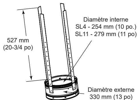
Stabilisateur de cheminée SL11/SL4
