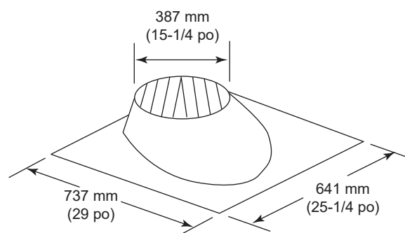
RF570 Solin de toit
