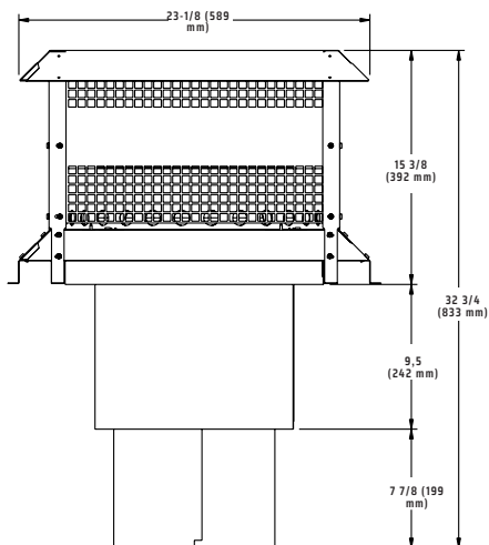
Chapeau de l'extrémité carré - ST1175/ST475
