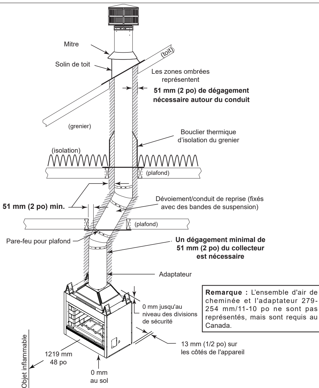
Figure 3.2 Dégagements par rapport aux matériaux inflammables
