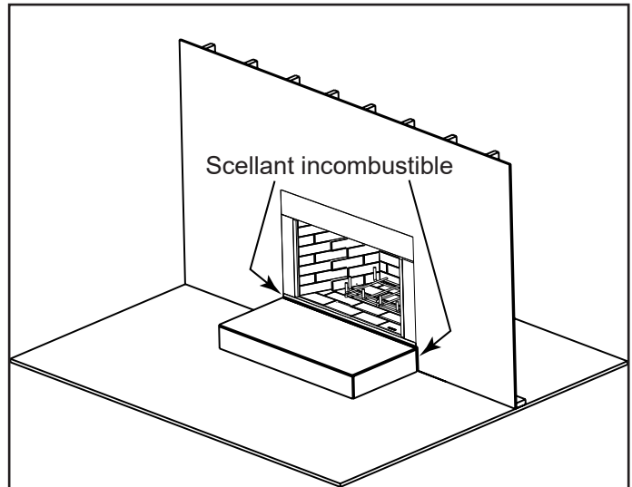
Figure 7.9 Placer le produit d'étanchéité incombustible
