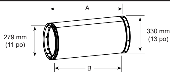
Sections de cheminée
