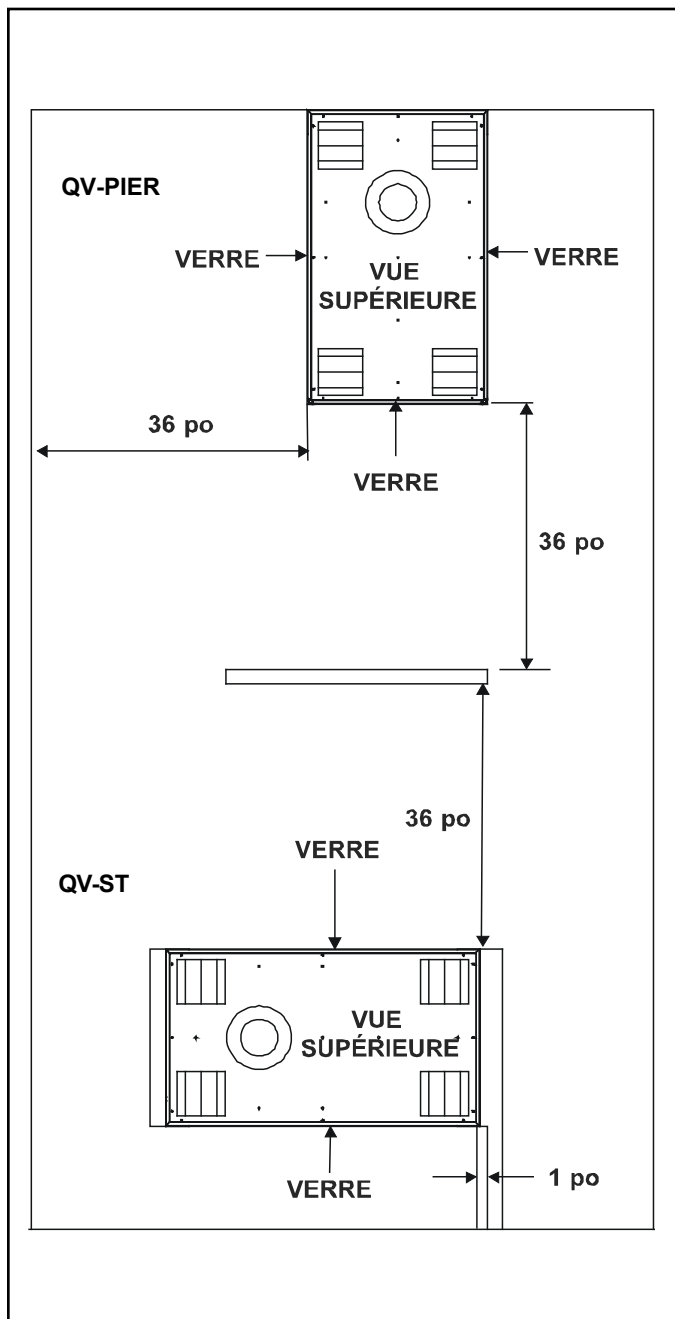
Figure 3. Dimensions du foyer, emplacements, et exigences en termes d'espace.
