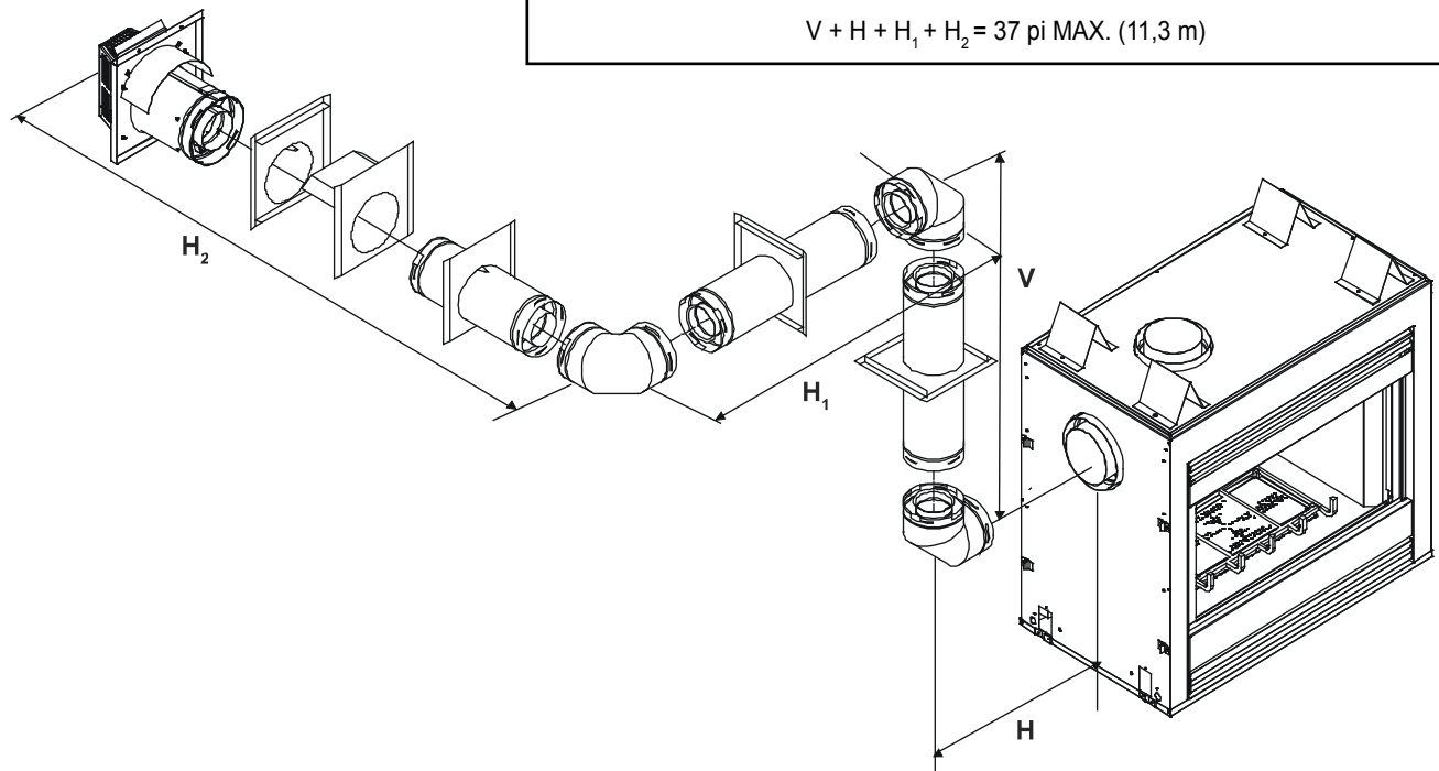
Figure 14. Évacuation avec trois coudes de 90°
