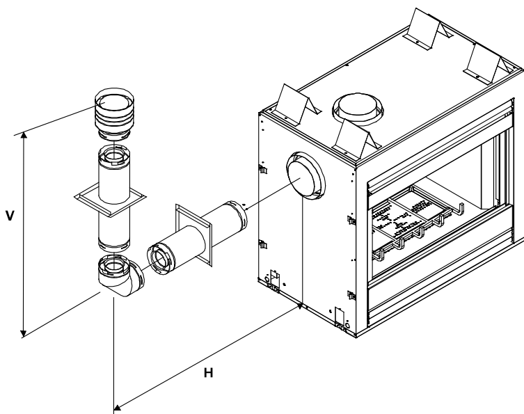
Figure 9. Évacuation avec un coude de 90°
