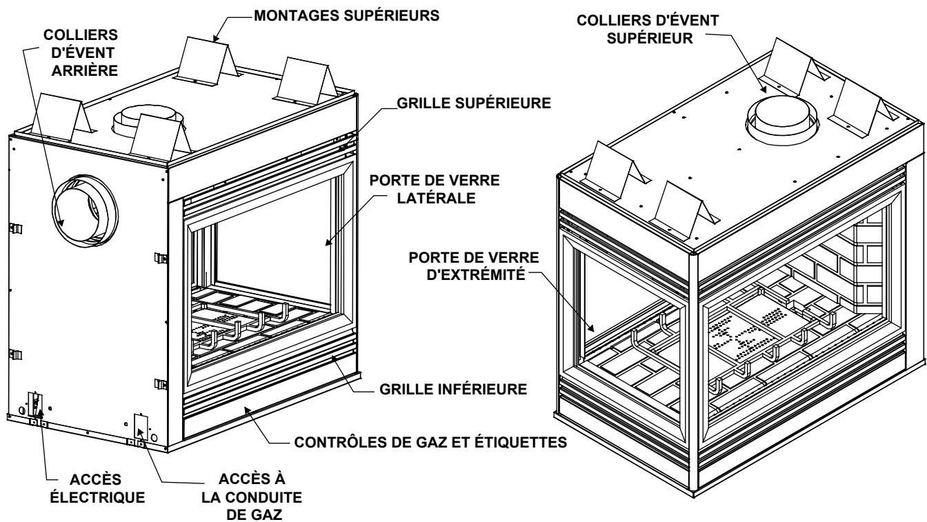
Figure 1. Diagramme de QV-PIER
