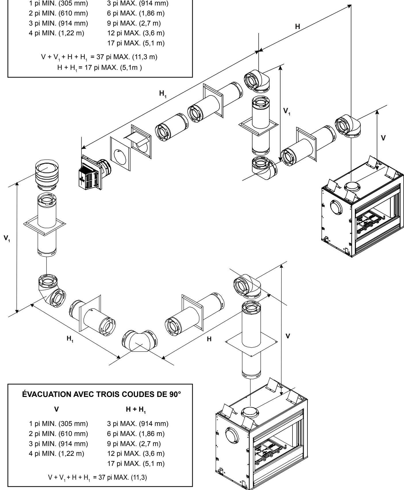
Figure 15. Évacuation avec trois coudes de 90°
