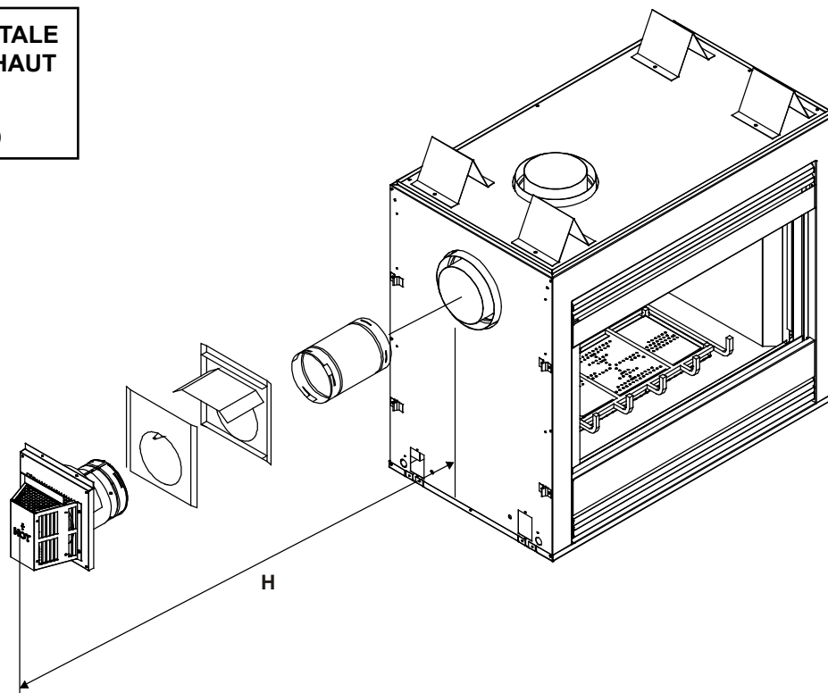
Figure 8. Évacuation horizontale tout droit vers l'extérieur
