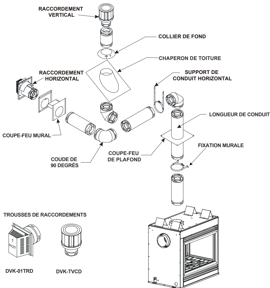
Figure 6. Composants du système d'évacuation et des trousse de raccordement
