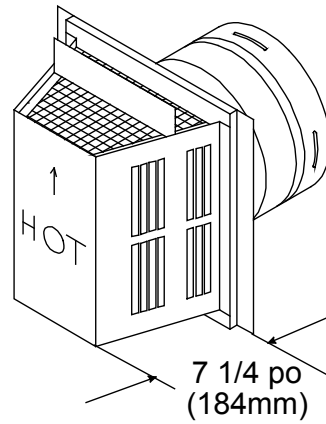
Figure 29. Raccordement à chapeau trapézoïde
