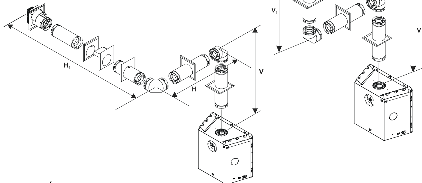
Figure 14. Évacuation avec deux coudes de 90°
