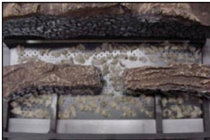
Figure 40. Placement du matériau de tison
