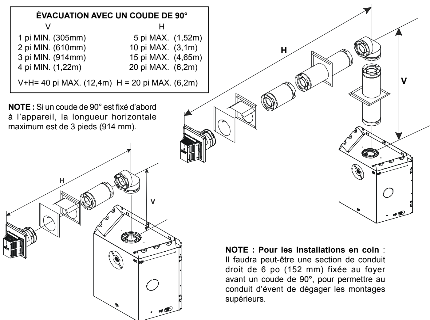
Figure 12. Évacuation avec un coude de 90°
