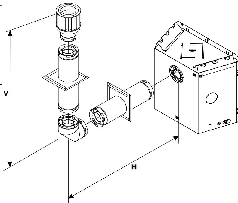
Figure 11. Évacuation avec un coude de 90°
