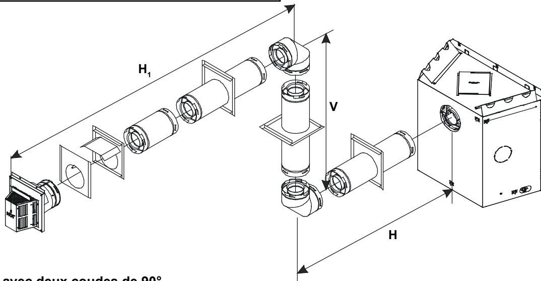
Figure 13. Évacuation avec deux coudes de 90°
