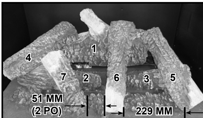
Figure 13 Mesure de placement des bûches
