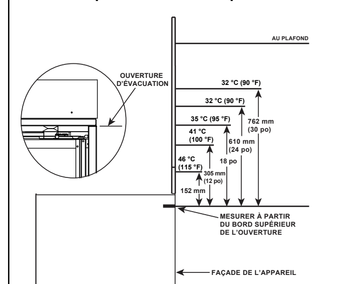
Figure 2.2 Températures de bonne foi à la surface du mur au-dessus de l'appareil avec ensemble de chaleur passive installé
