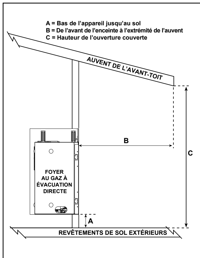
Figure 3.6 Applications extérieures protégées - Dimensions
