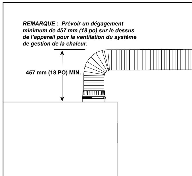
Figure 3.5 Dégagement pour le système de gestion de la chaleur
