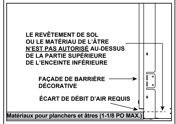
Figure 10.3 Écart de débit d'air requis
