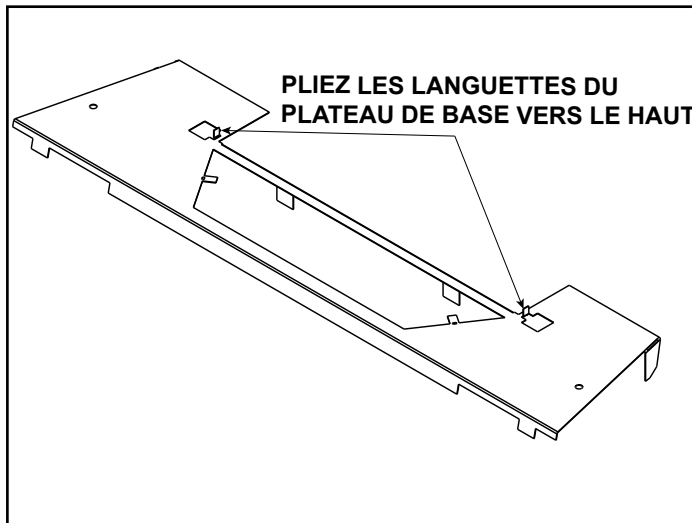
Figure 2 Pliez la languette du plateau de base - CAL36X-SG/WB uniquement
