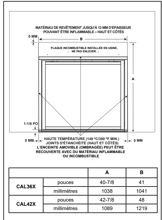
Figure 10.2 Schéma du revêtement incombustible
