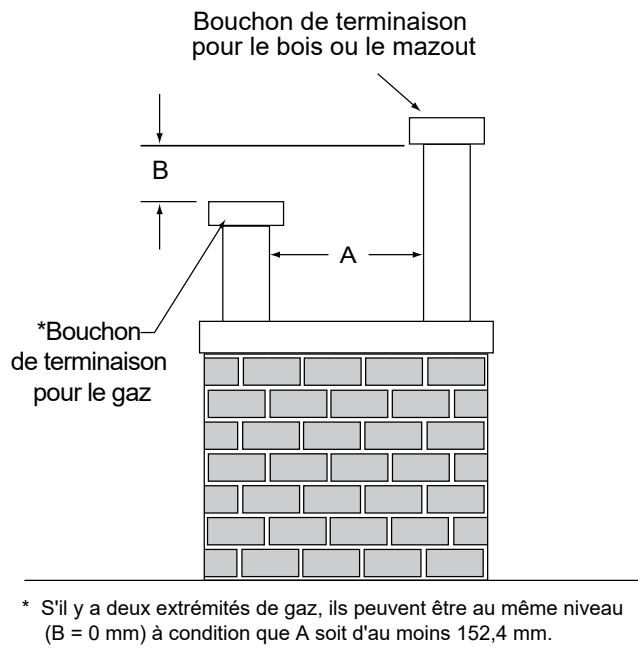
Figure 4.2 Chapeaux des extrémités décalés
