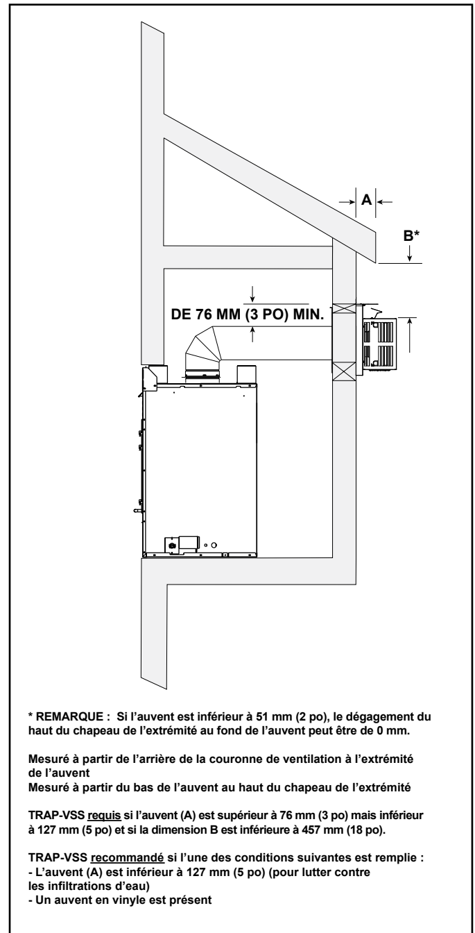
Figure 3.13 Enchâssure extérieure - Exigences minimales de hauteur
