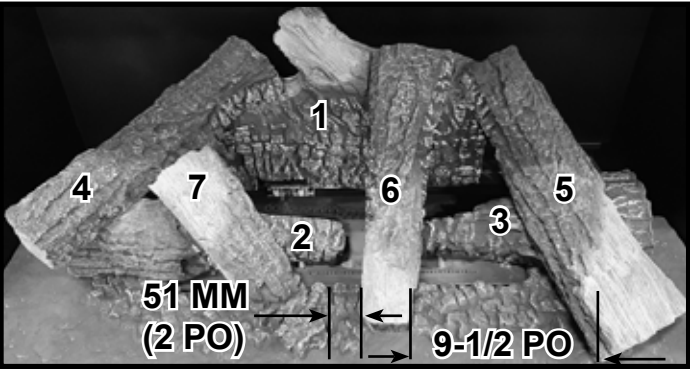
Figure 13 Mesure de placement des bûches
