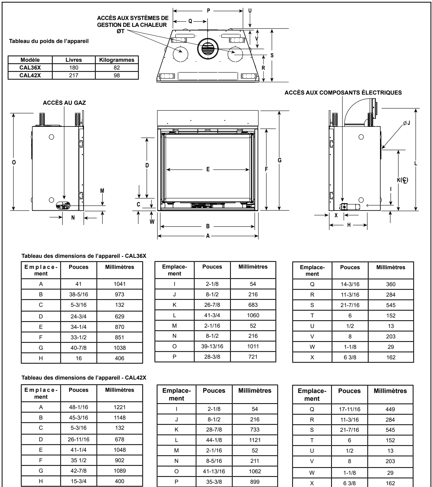
Figure 3.1 Dimensions de l'appareil CAL36X, CAL42X
