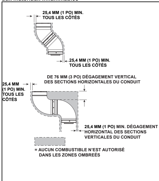
Figure 5.3 Dégagements entre l'évent et les matériaux de charpente combustibles
