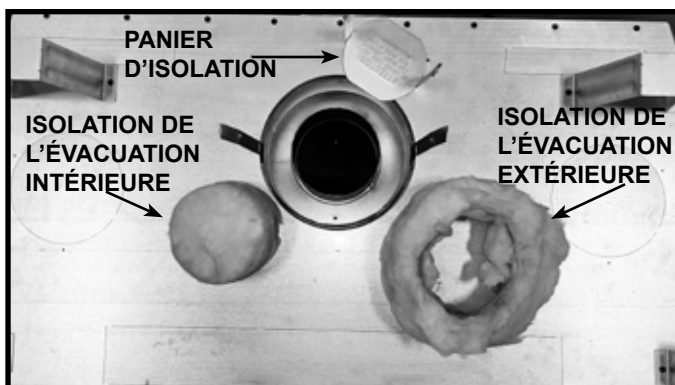
Figure 6.5 Retirer le panier d'isolation, l'isolation de l'évacuation intérieure et l'isolation de l'évacuation extérieure
