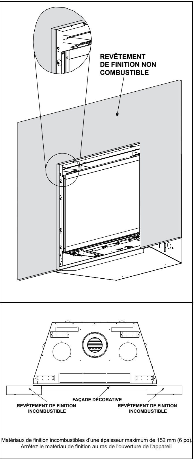
Figure 10.11 Méthode d’ajustement intérieur
