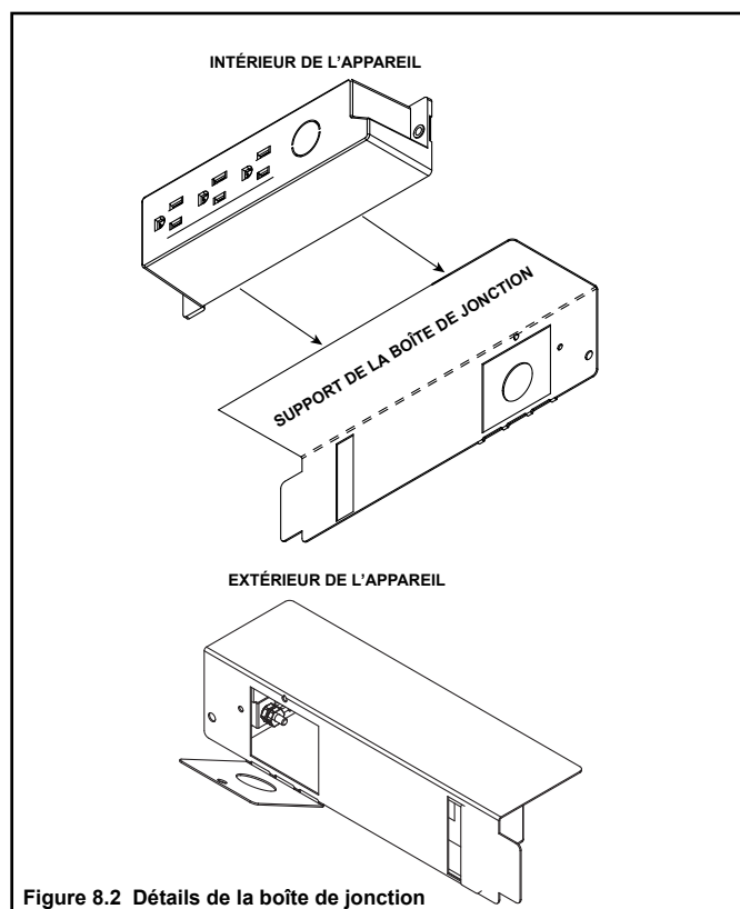
Figure 8.2 Détails de la boîte de jonction
