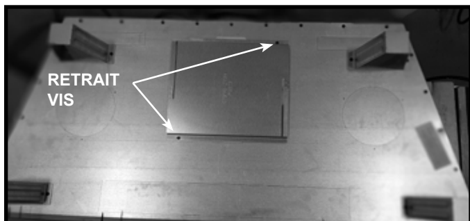
Figure 6.1 Retirer l'écran thermique coudé en enlevant les deux vis
