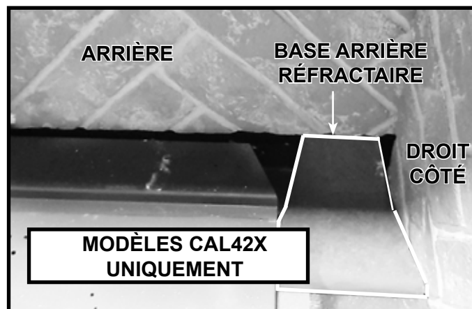
Figure 11.7 Modèles CAL42X uniquement : Pièce réfractaire de la base arrière installée (côté droit illustré)
