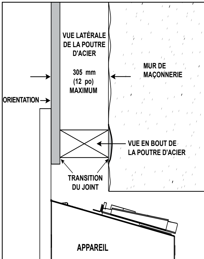
Figure 3.14 Détails sur l'étanchéité de transition pour les extensions murales (vue latérale)
