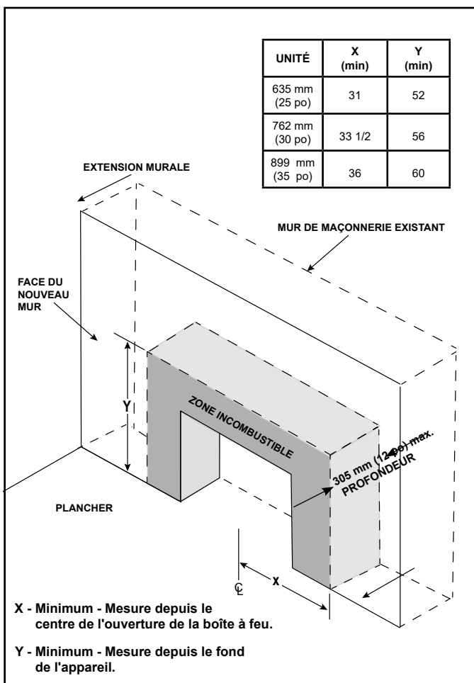
Figure 3.11 Exigence d'encadrement incombustible
