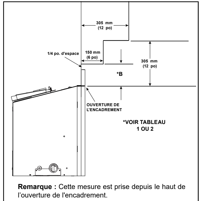
Figure 3.16 Dimensions verticales minimales et horizontales maximales - Incombustible
