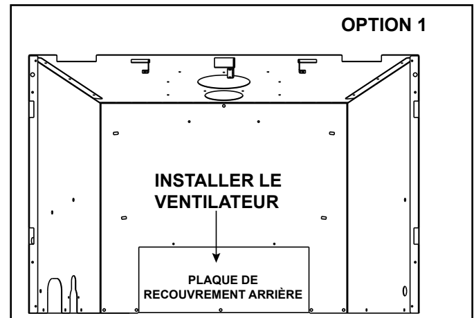
Figure 6.4 Couvercle retiré (Option 1)
