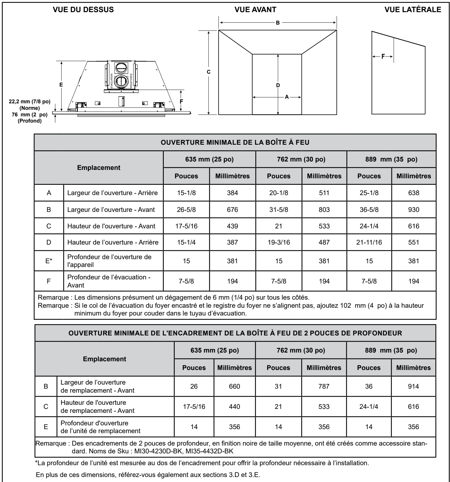
Figure 3.10 Ouverture de la boîte à feu - Encadrement régulier - 19 mm (3/4 po)
