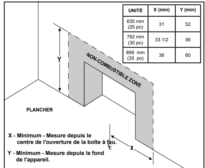
Figure 3.12 Exigence du revêtement incombustible
