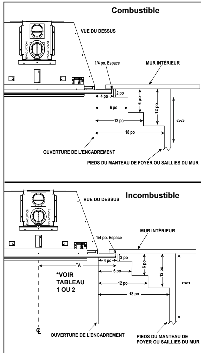
Figure 3.15 Dégagements par rapport aux pieds du manteau de foyer ou saillies du mur (acceptables des deux côtés de l'ouverture de l'encadrement).
