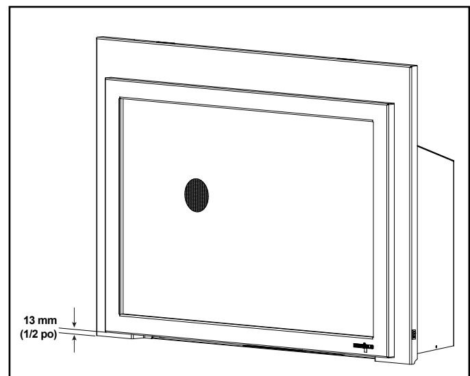
Figure 3.9 Minimum requis de 12,7 mm (1/2 po). Espace
