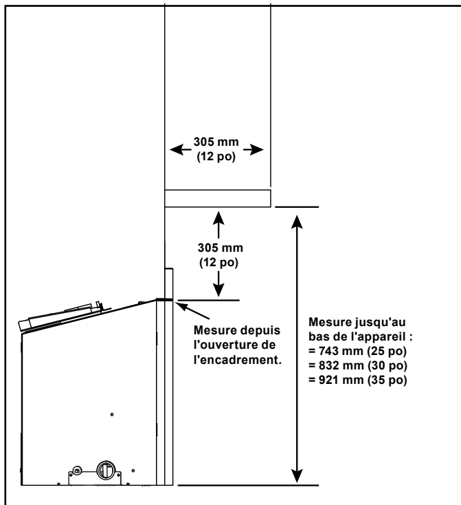
Figure 3.17 Dimensions verticales minimales et horizontales maximales - Combustible
