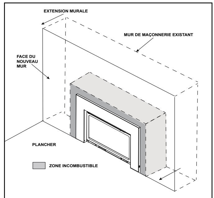
Figure 3.13 Exigence du revêtement / encadrement incombustible
