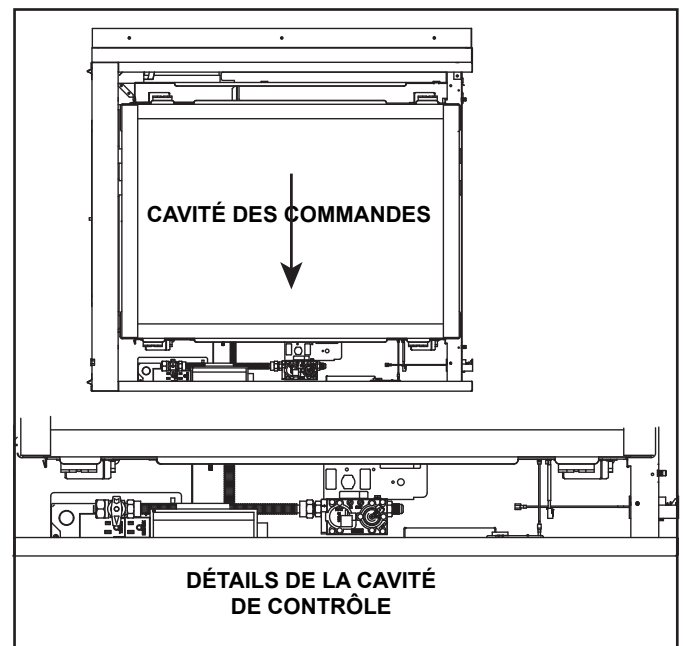
3.5 Emplacement de la cavité de contrôle (PIER-36TRB-IFT Montré)
