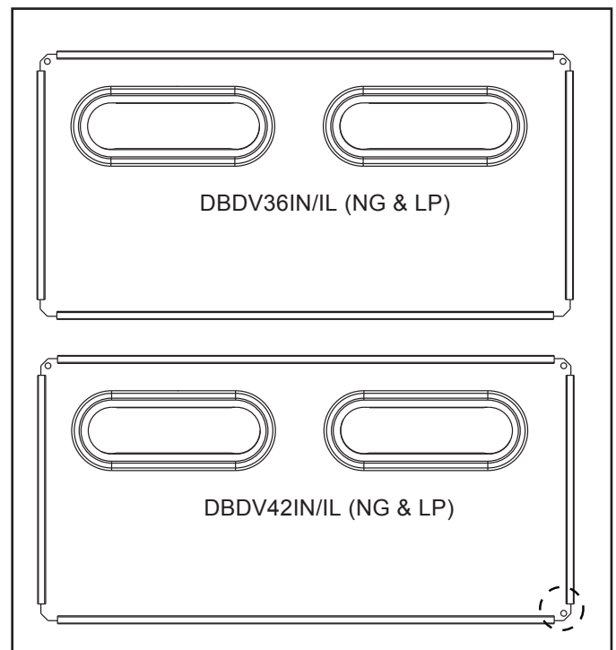
Figure 4.3 - Exemple d'identification du brûleur
