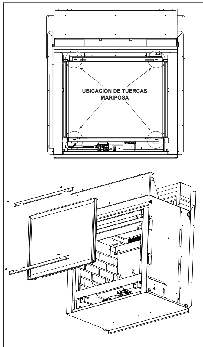
9.1 Conjunto de vidrio - Lado interior
