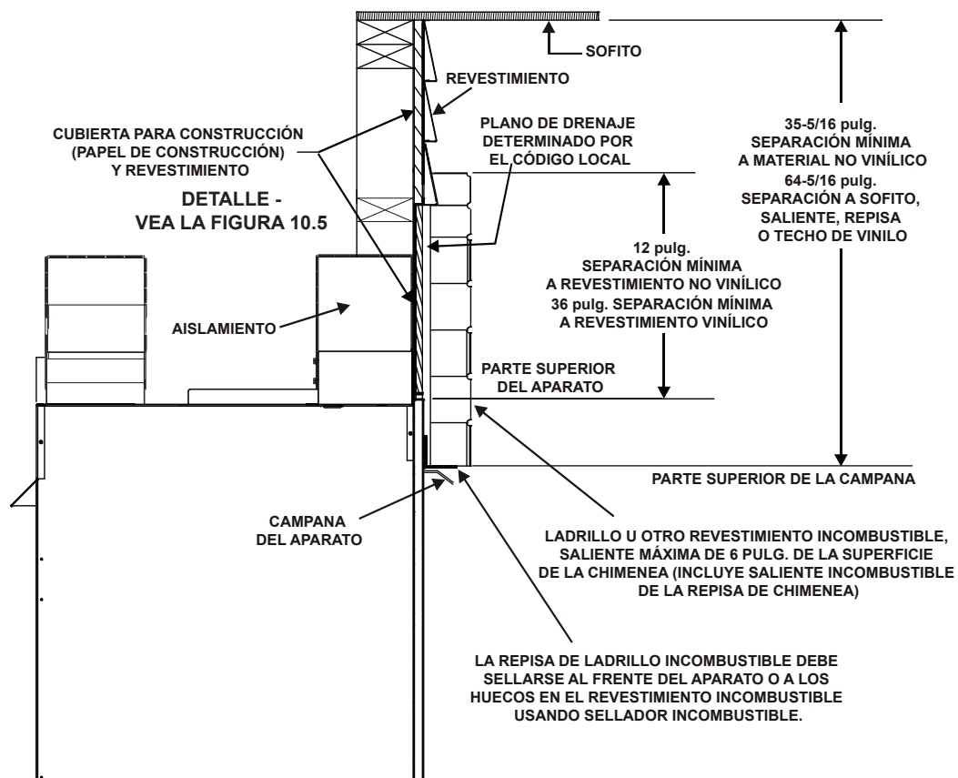
Figura 8.12 Vista exterior con material de revestimiento incombustible
