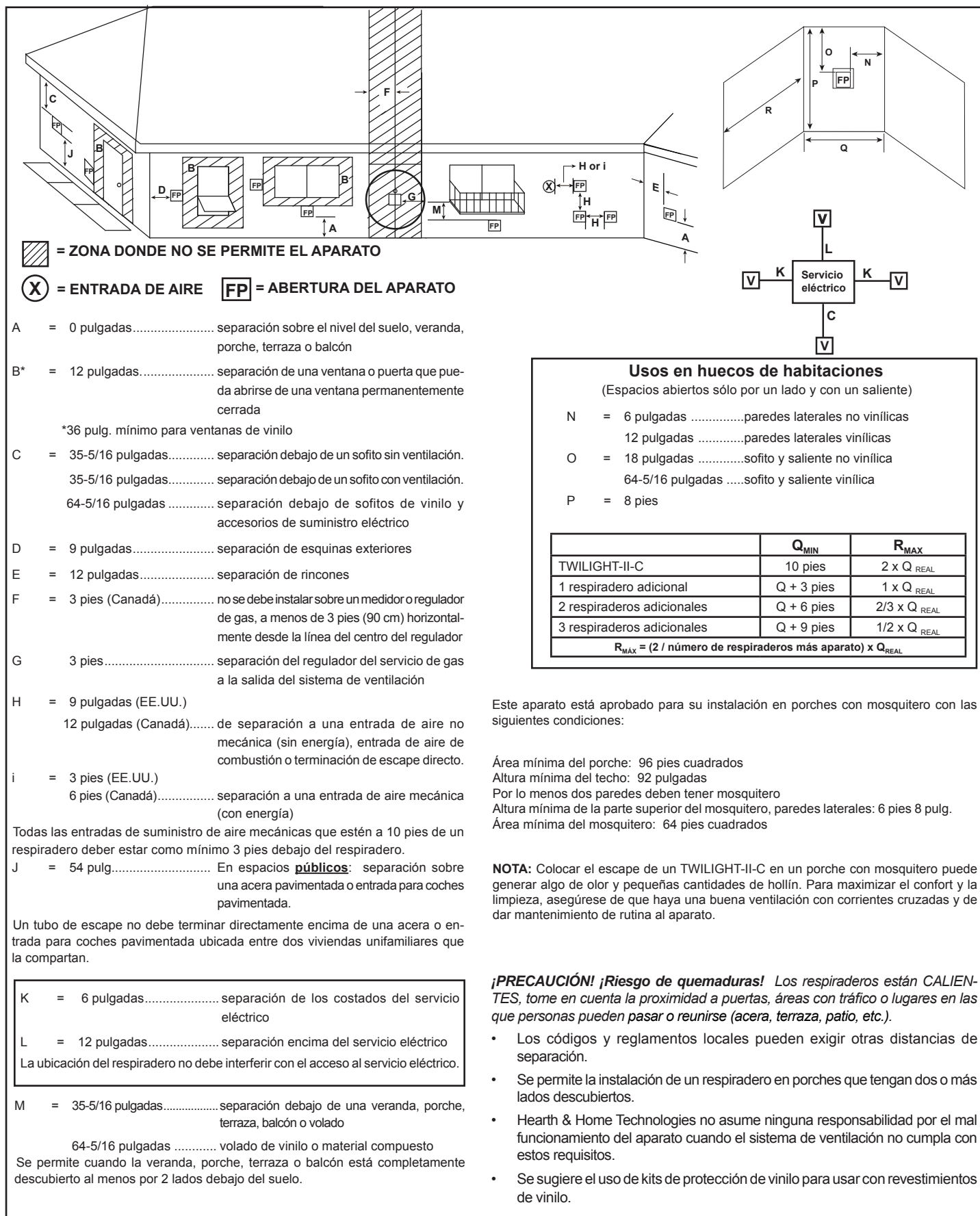
Figura 4.1 Distancias mínimas de separación de la terminación
