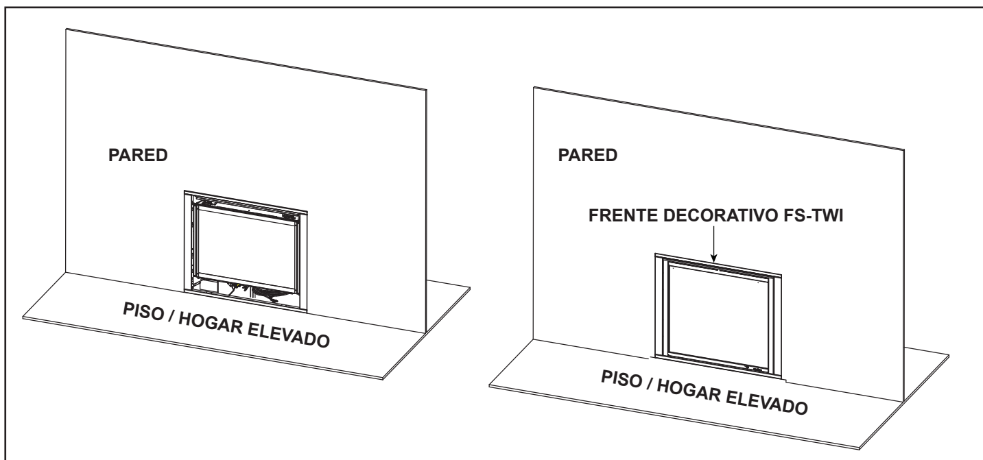
Figura 8.4 Aparato instalado en el piso o en un hogar elevado
