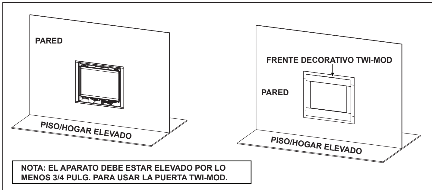
Figura 8.5 Aparato instalado separado del piso
