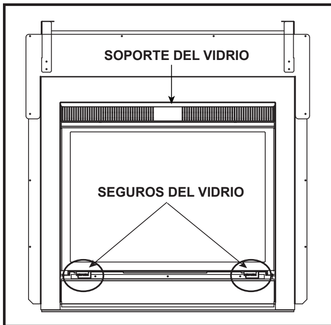
9.3 Ubicación de los seguros del vidrio - Lado exterior
