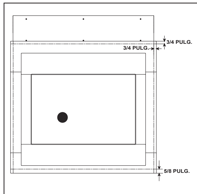
Figura 8.3 Frente decorativo sobrepuesto al marco decorativo
