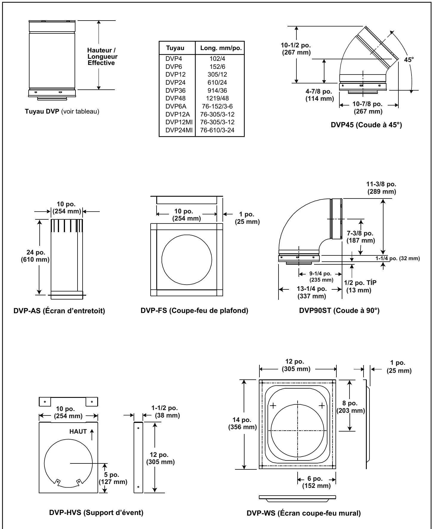
Figure 16.2 Composants d'évents DVP*
