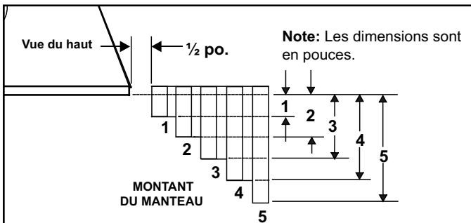
Figure 11.2 Dégagements aux montants du manteau ou aux projections murales (Valables des deux côtés de l'ouverture.)
