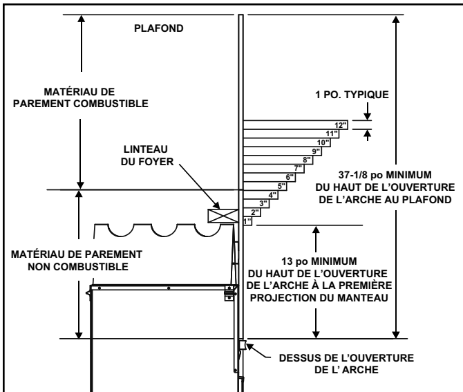
Figure 11.1 Dégagements au manteau ou autres matériaux combustibles au-dessus de l'appareil
