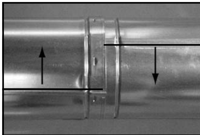
Figure 8.11 Pivotez les joints pour le démontage
