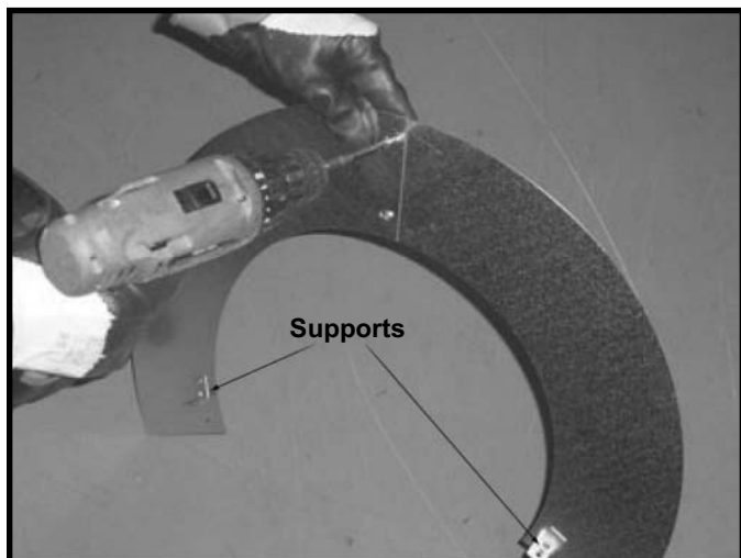
Figure 8.16 Assemblage de la mitre
