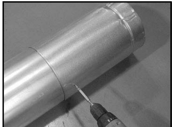
Figure 8.8 Vis dans la section coulissante
