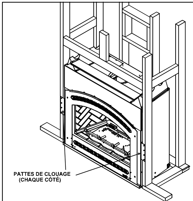
Figure 7.3 Placement, nivelage et fixation appropriés de l'appareil
