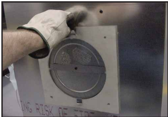
Figure 9.6 Repliez les pattes vers le centre du capuchon plombé (90°) et retirez le panier d'isolant.
