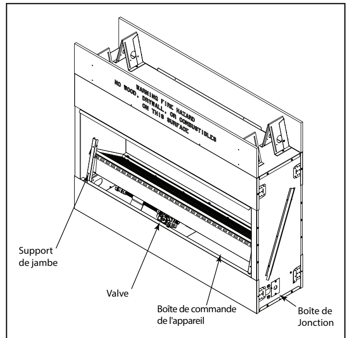
Figure 5.1. Appareil avec moteur levé
