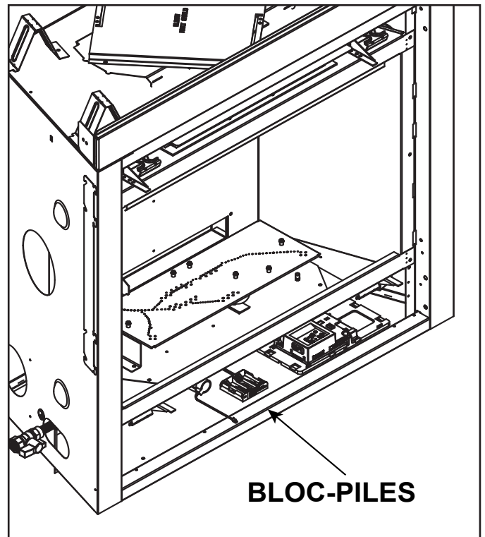
3.5 BLOC-PILES SITUÉ DANS LA CAVITÉ DES COMMANDES
