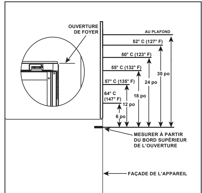
Figure 3.3 Températures de la surface du mur au-dessus de l'appareil
