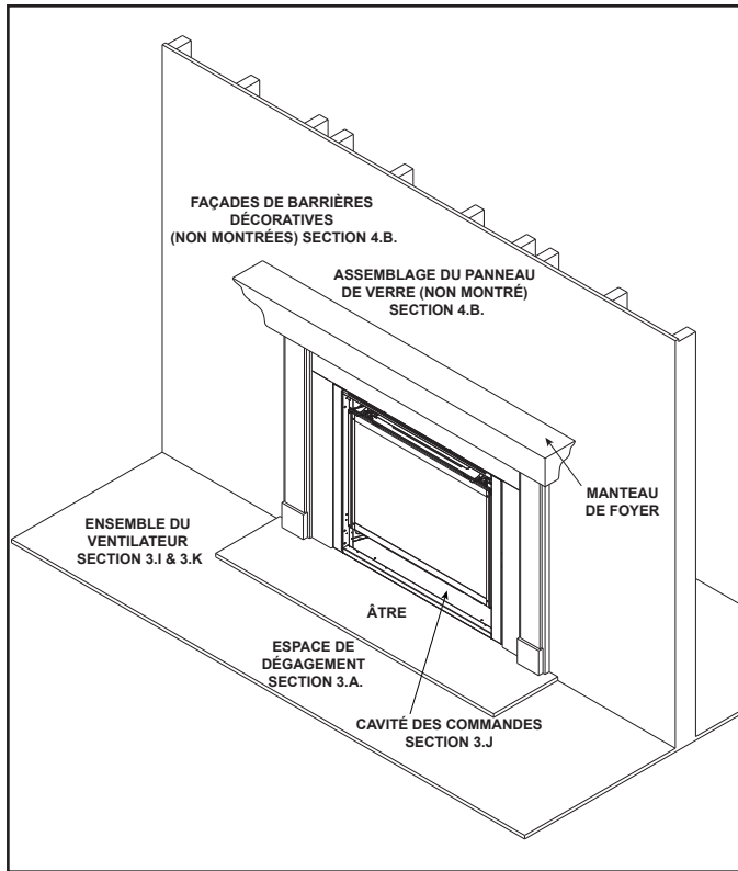
Figure 3.2 Pièces générales d'utilisation
