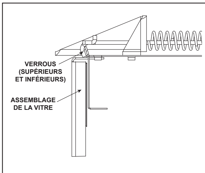
Figure 4.1 Panneau de verre fixe
