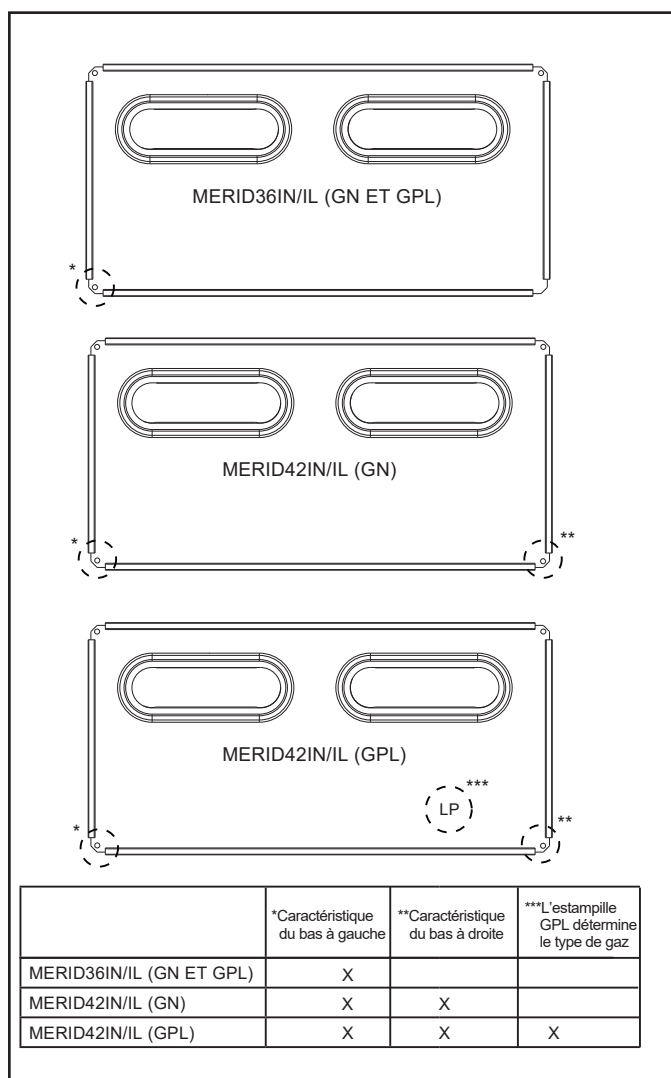
Figure 4.3 - Exemple d'identification du brûleur
