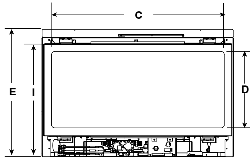
VUE DE L'AVANT
