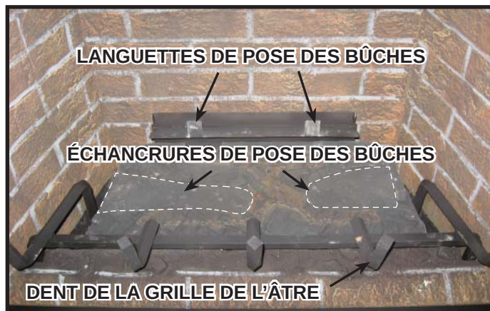
Figure 2 Languettes de pose des bûches
