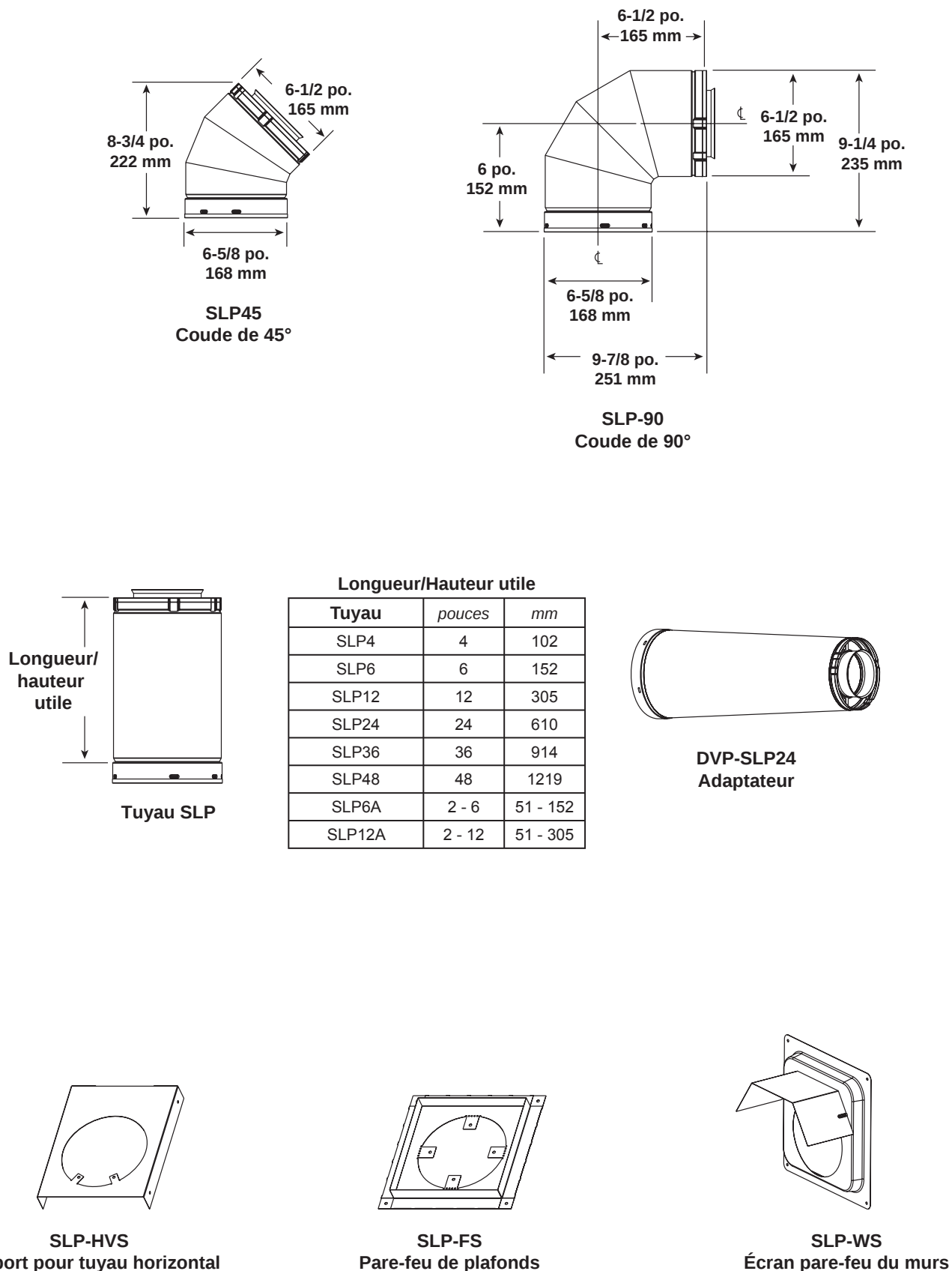
Figure 16.8 Composants du conduit d'évacuation de la série SLP
