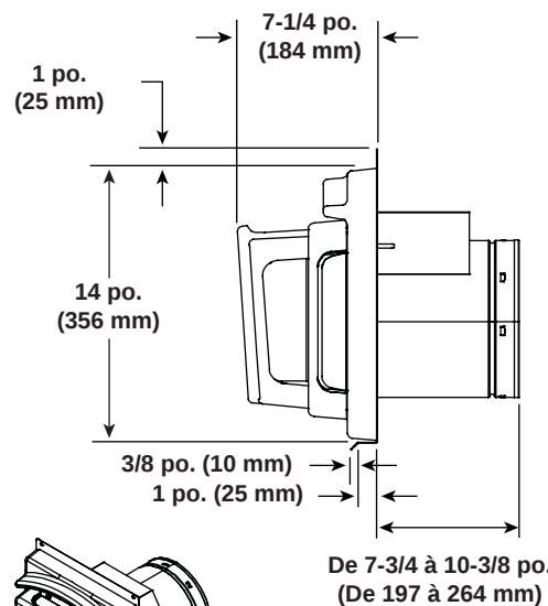
DVP-FBHT Capuchon de brique réfractaire
