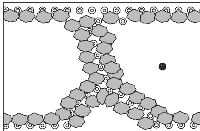
Figure 14.10 Braises recouvrant partiellement les orifices du brûleur (propane seulement)
