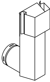
SLK-SNKD Schacht-Mündungselement
