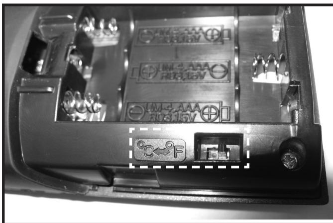
Abbildung 12.5 Temperaturskala
