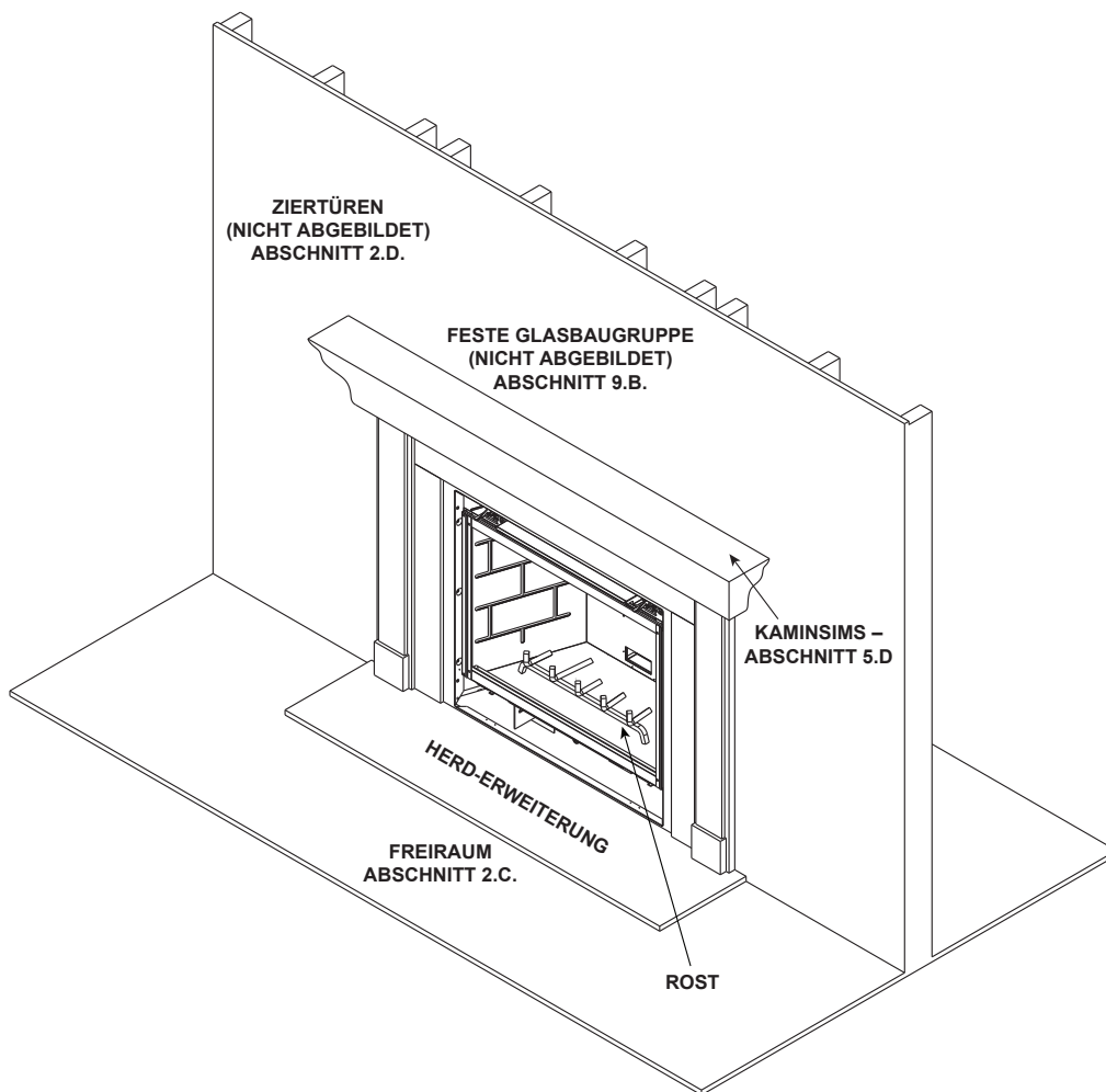
Abbildung 2.1 Allgemeine Funktionsteile
