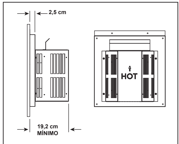
Figura 10.15 Respiradero
