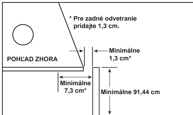
Obr. 5.5 Vzdialenosti od bočnej rímky alebo výčnelkov steny (prípustné na oboch stranách otvoru).
