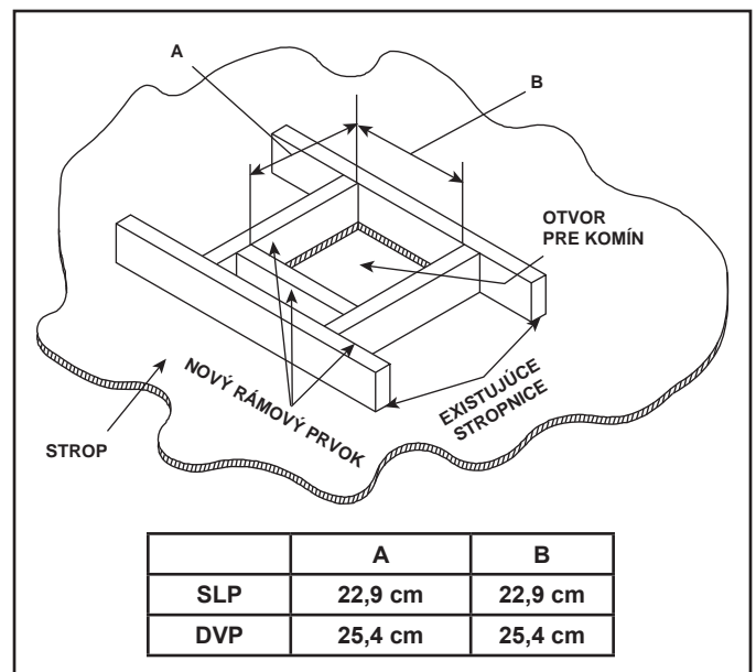
Obr. 10.14 Otvor a nové rámové prvky
