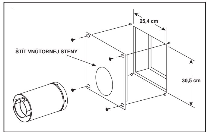
Obr. 10.13 Rúra dymovodu a požiarna zábrana
