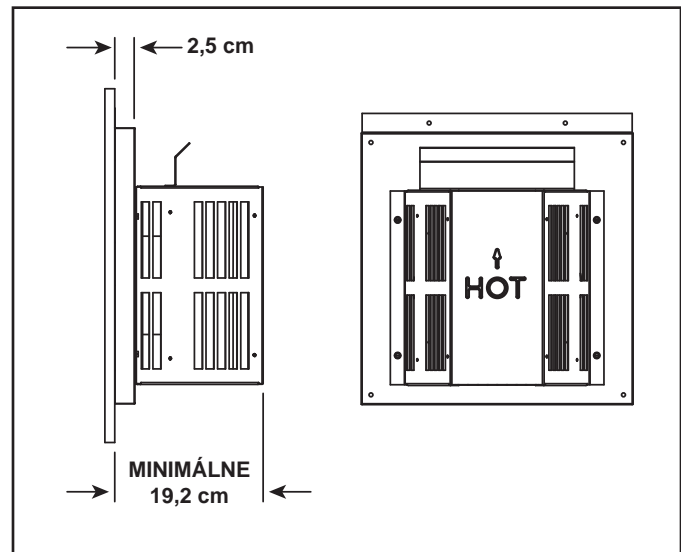
Obr. 10.18 Kryt vývodu
