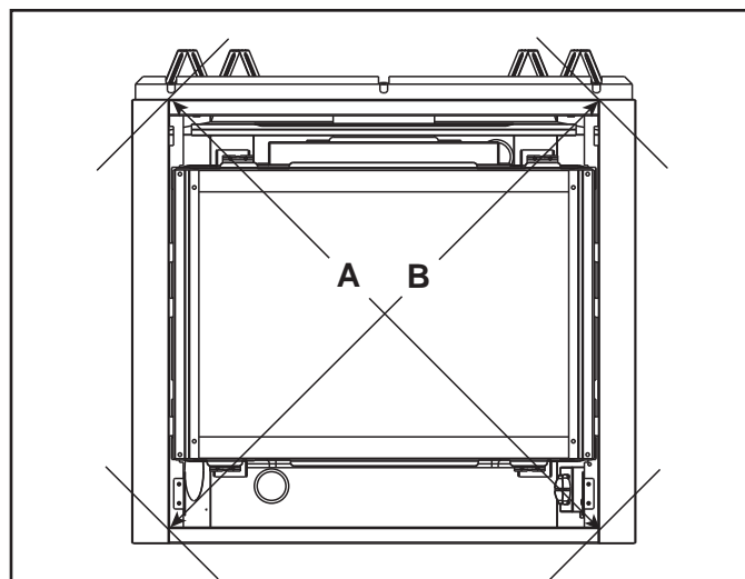
Obr. 9.15 Umiestnenie krbu do štvorca
