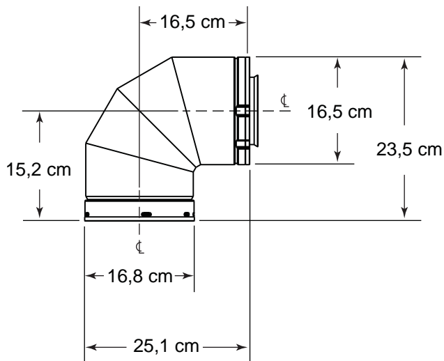
SLP-90 – 90° koleno
