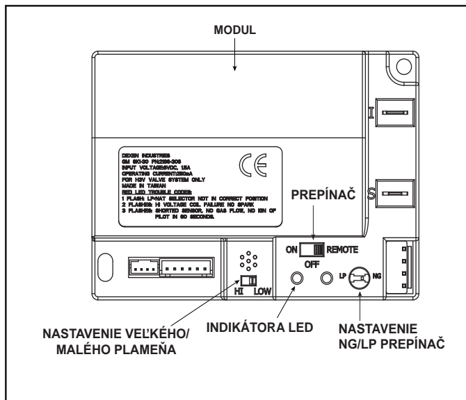
Obr. 2.3 Ovládací modul
